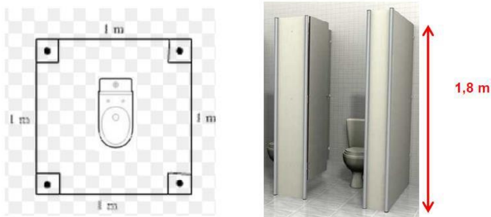
Figura 6 - Dimensões mínimas de sanitários a serem adotadas no canteiro.
