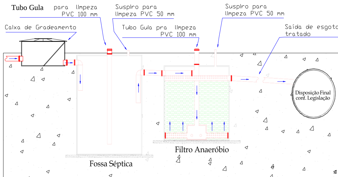
Figura 13 - Modelo de Sumidouro a ser utilizado na implantação do Canteiro de Obras (SE)
