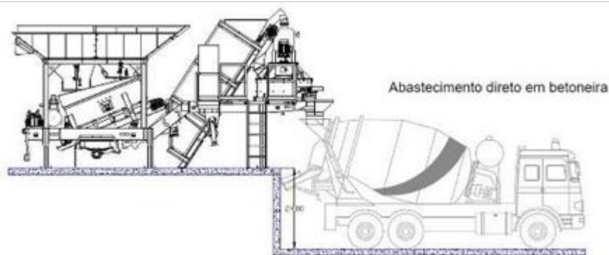
Figura 10 – Esquemático da usina móvel de concreto
