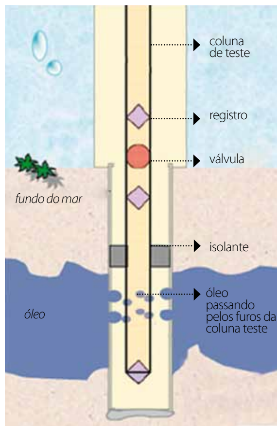
Fig.11 - Esquema do teste de formação.
