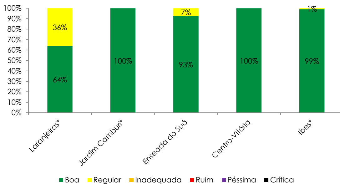
Gráfico 6.11 - Índice de qualidade do ar com base no poluente PTS nas estações da RAMQAr.
