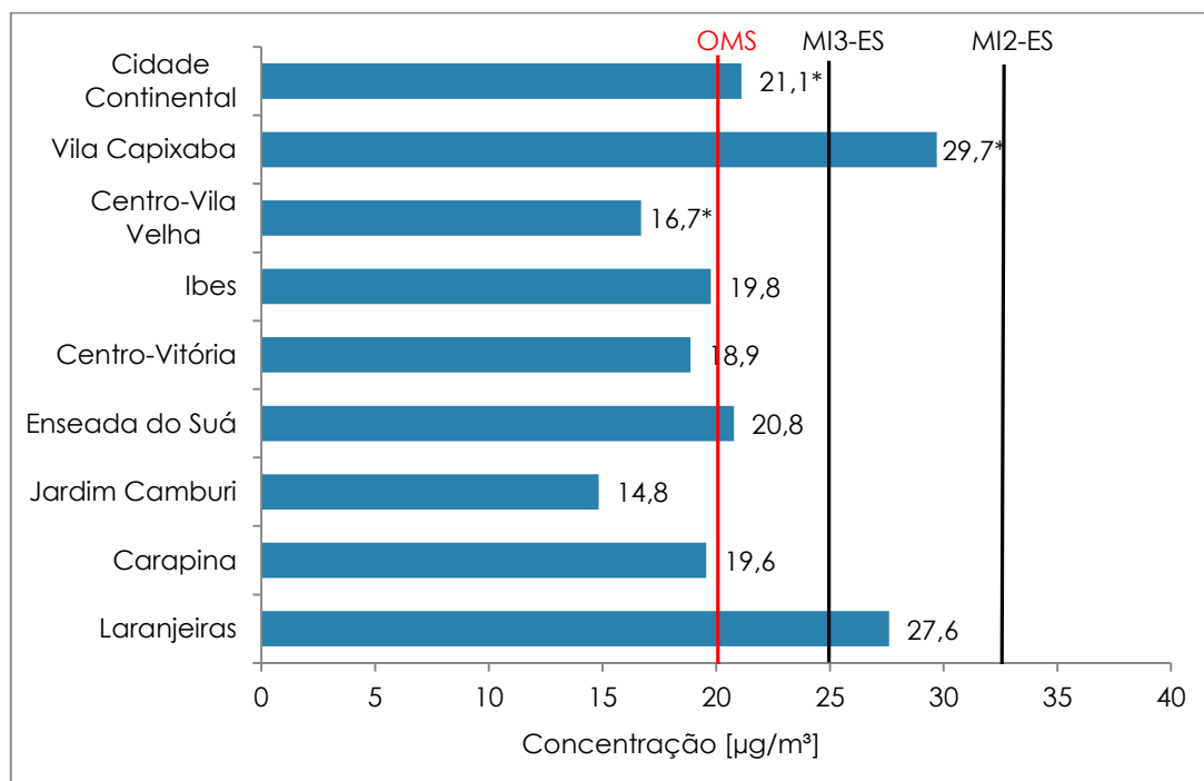
Gráfico 6.5 - Concentração média anual de PM 10 nas estações da RAMQAr.
