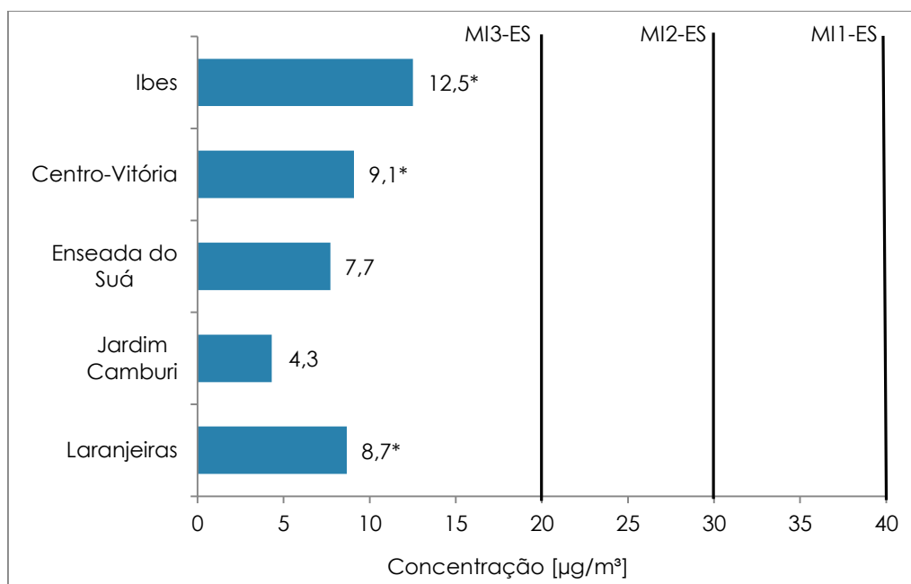
Gráfico 6.17 - Concentração média anual de SO 2 nas estações da RAMQAr.
