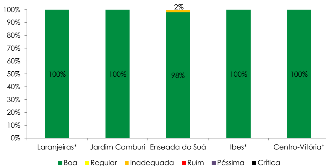
Gráfico 6.18 - Índice de qualidade do ar com referência ao poluente SO 2 nas estações da RAMQAr.
