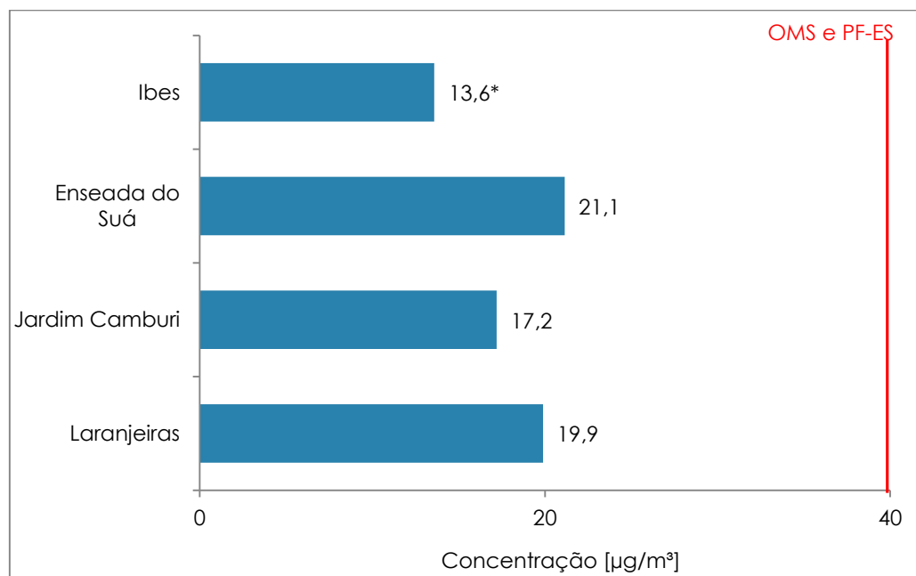
Gráfico 6.22 - Concentrações médias anuais de NO 2 nas estações da RAMQAr.
