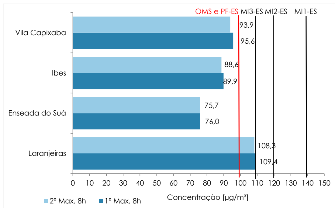
Gráfico 6.26 - Concentração média 8h máxima de O 3 nas estações da RAMQAr.
