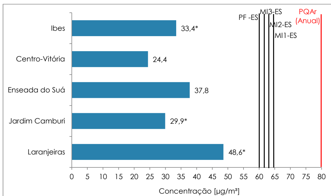
Gráfico 6.10 - Concentração média anual de PTS nas estações da RAMQAr.
