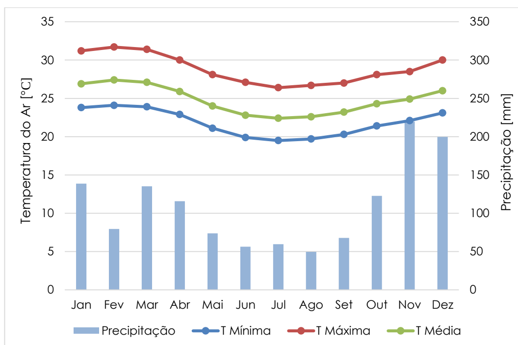
Gráfico 2.1- Normais climatológicas da estação Vitória (Temperatura e Precipitação) – 1981 - 2010
