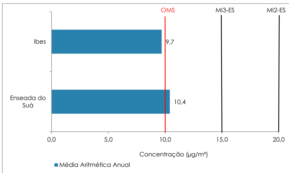
Gráfico 6.2 - Concentração média anual de PM 2,5 nas estações da RAMQAr.
