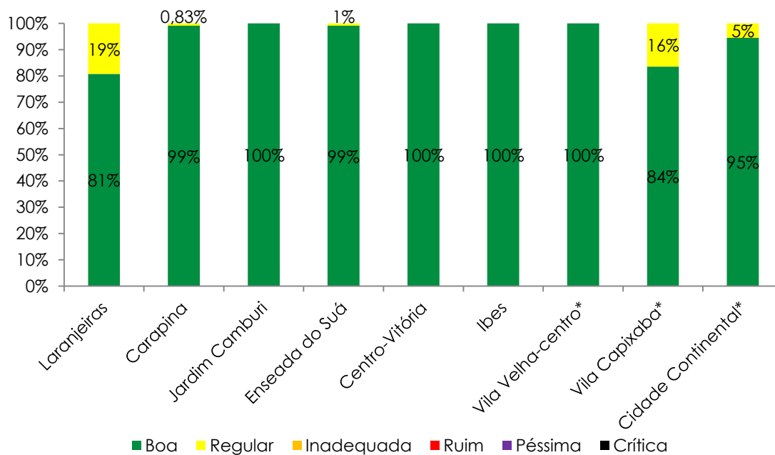
Gráfico 6.6 - Índice de qualidade do ar com referência ao poluente PM_{10} nas estações da RAMQAr.
