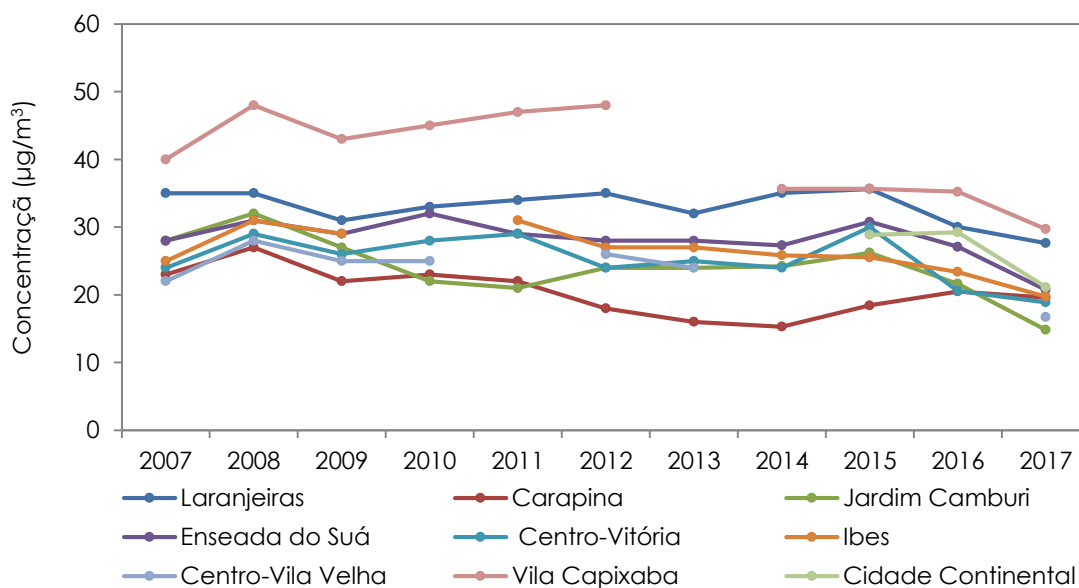
Gráfico 6.8 - Séries temporais das concentrações médias anuais de PM 10 nas estações da RAMQAr.
