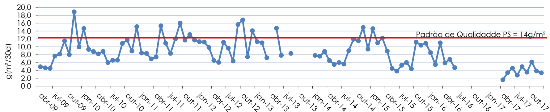
Gráfico 6.15 - Série temporal da taxa de deposição de partículas para o período de abril de 2009 a dezembro de 2017 para as estações da RMPS.
