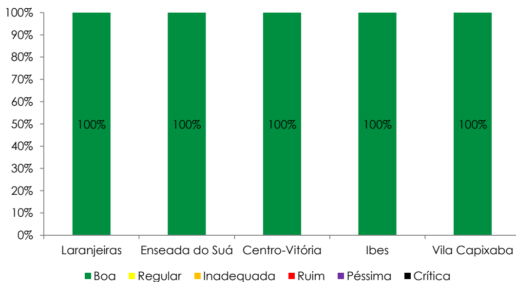
Gráfico 6.34 - Índice de qualidade do ar com referência ao poluente CO nas estações da RAMQAr.
