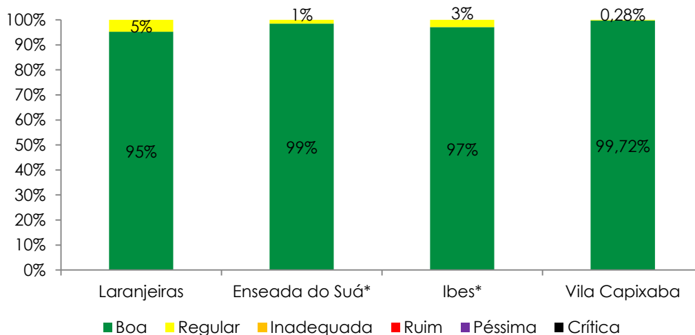
Gráfico 6.28 - Índice de qualidade do ar com referência ao poluente O 3 nas estações da RAMQAr.
