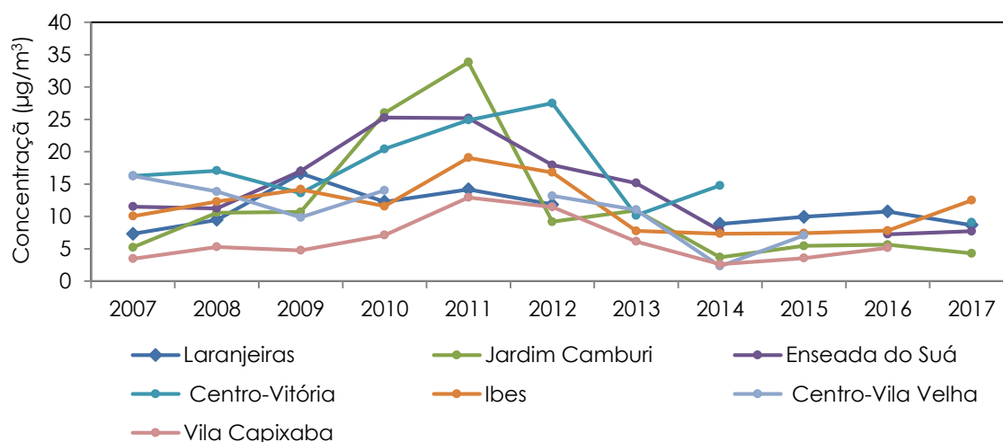
Gráfico 6.20 - Séries temporais das concentrações médias anuais de SO 2 nas estações da RAMQAr.
