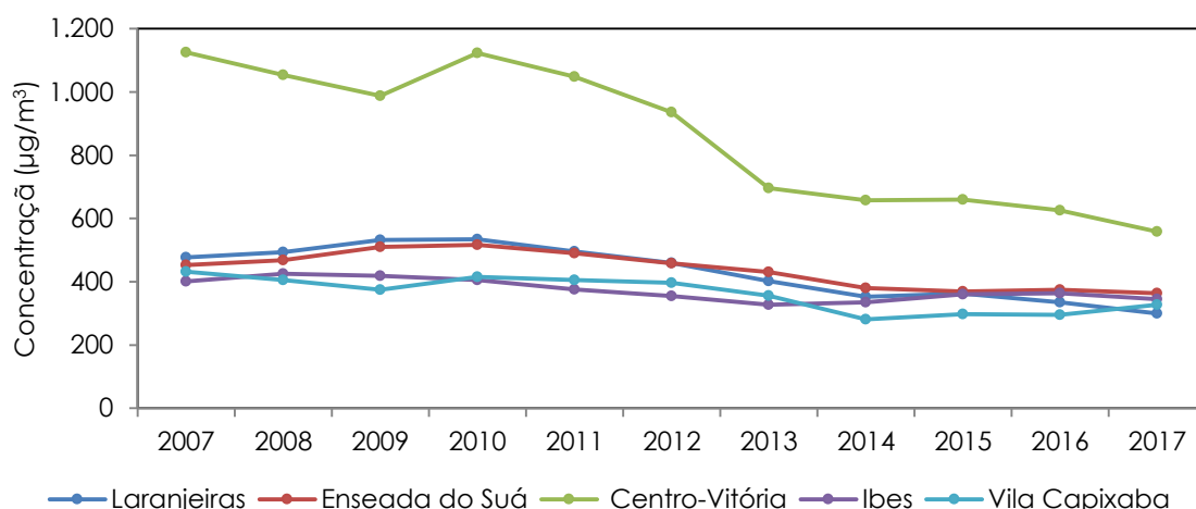
Gráfico 6.36 - Séries temporais das concentrações médias anuais de CO nas estações da RAMQAr.
