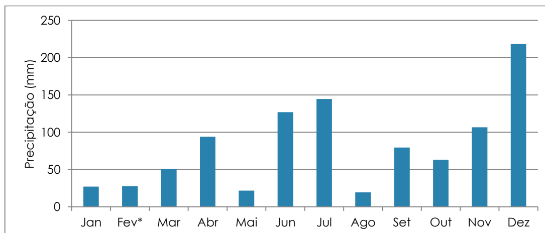
Gráfico 5.1 - Precipitação acumulada mensal na estação RAMQAr 2 - Carapina.
