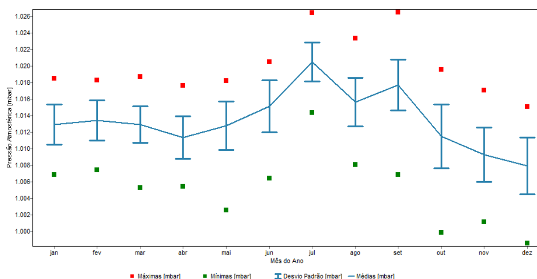
Gráfico 5.4 - Pressão atmosférica média mensal, máxima e mínima na estação RAMQAr 2 - Carapina.
