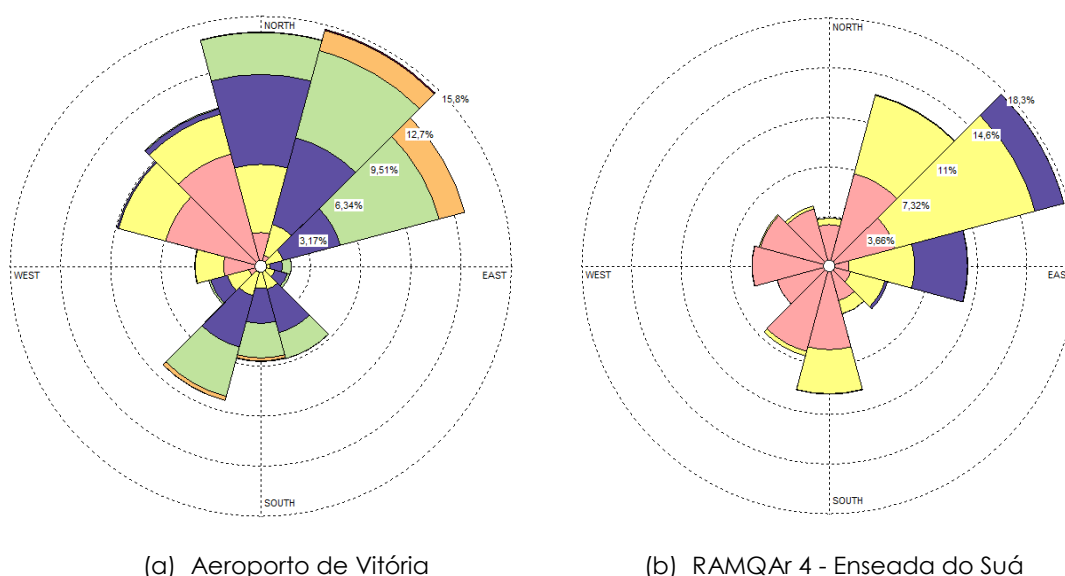
Gráfico 5.10 - Rosa dos ventos anual da RMGV.
