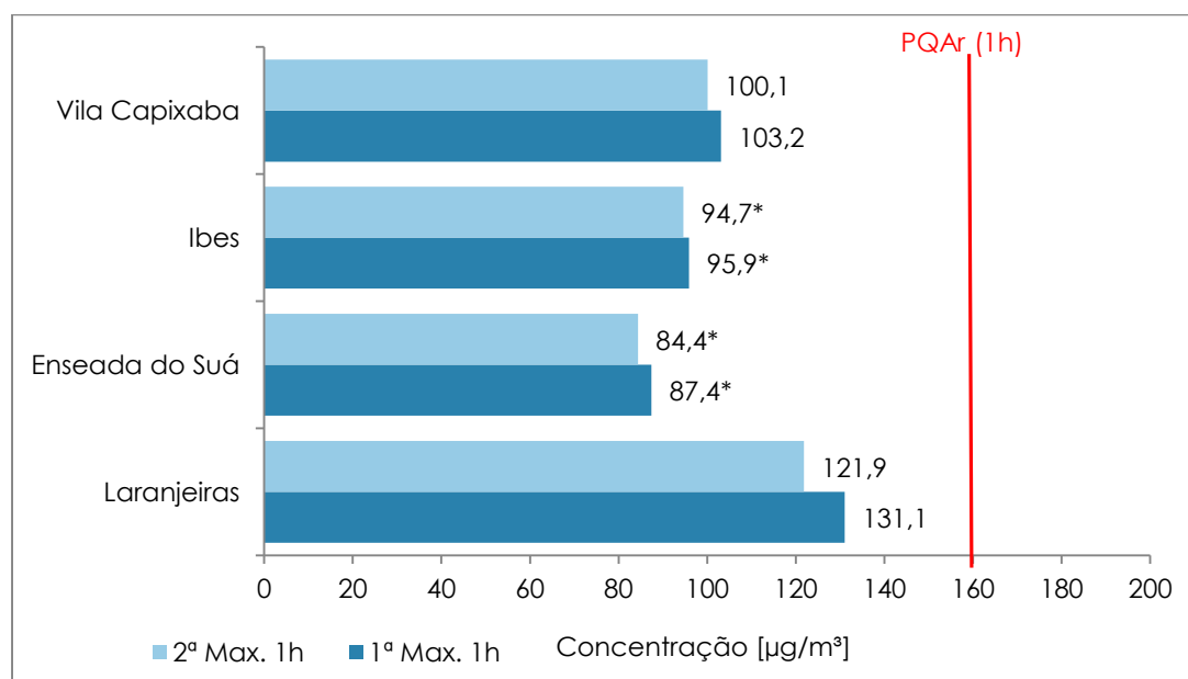
Gráfico 6.27 - Concentração horária máxima de O 3 nas estações da RAMQAr.
