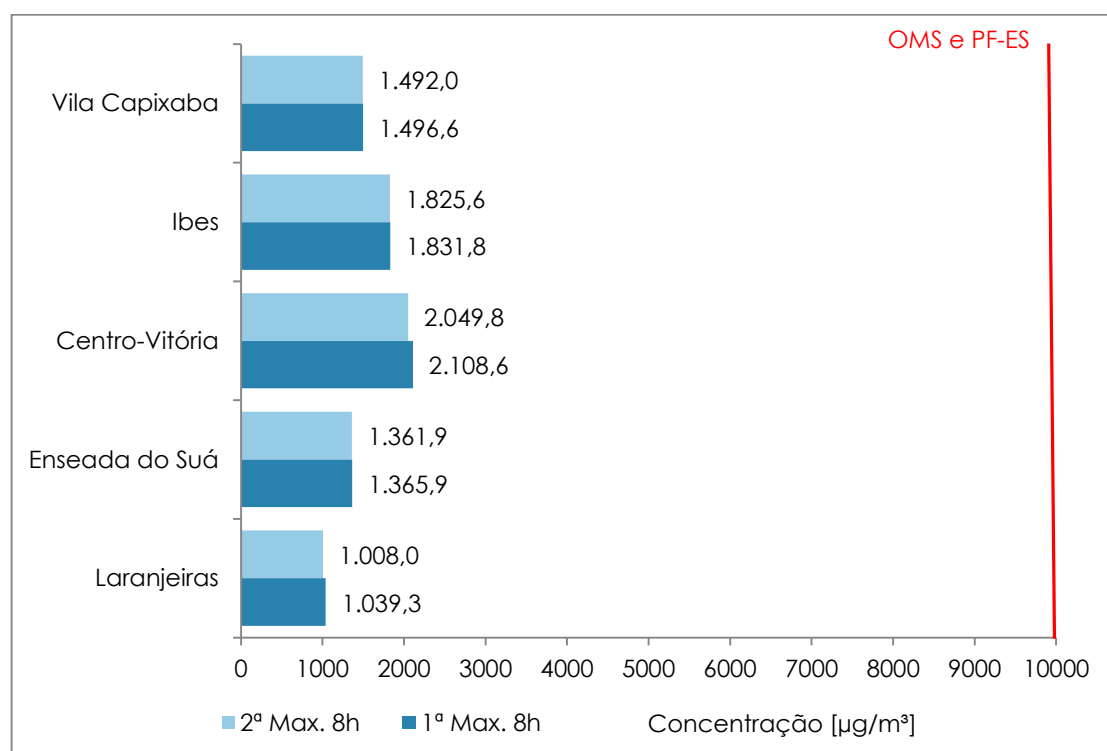
Gráfico 6.32 - Concentração média de 8h máxima de CO nas estações da RAMQAr.
