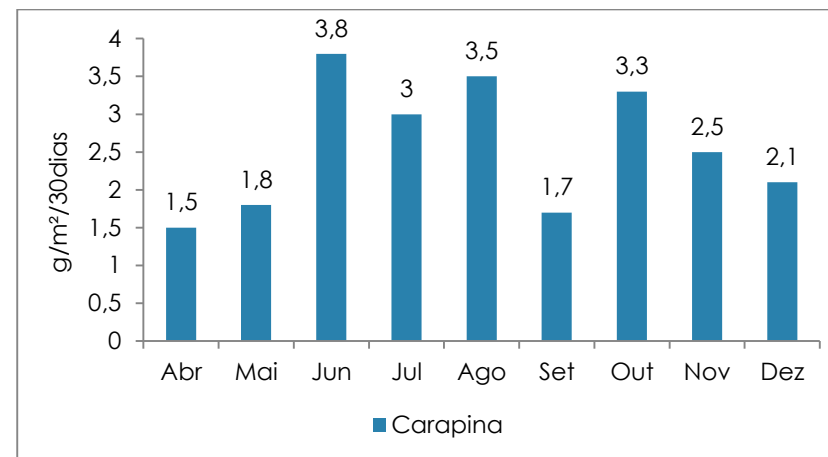
Gráfico 6.14 - Taxa de deposição de partículas ( \text{g/m}^2/30 dias) nas estações de monitoramento de para o ano de 2017.
