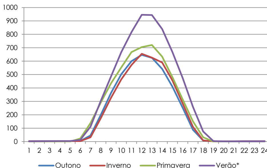
Gráfico 5.5 - Radiação solar média horária nos períodos de solstício e equinócio do ano na estação RAMQAr 2 - Carapina.
