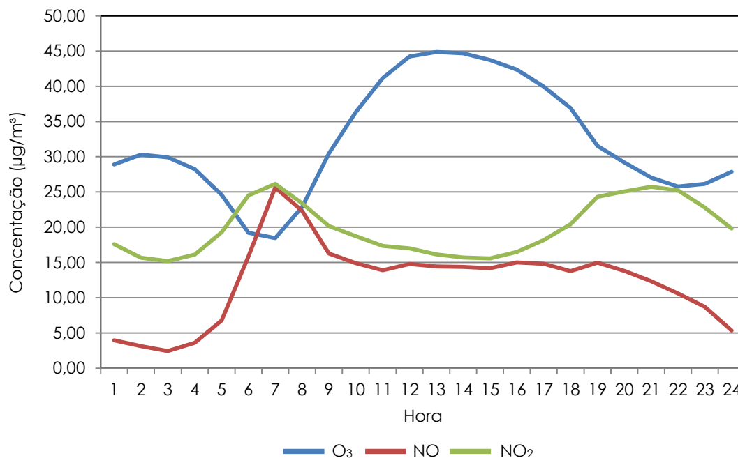
Gráfico 6.30 - Evolução horária dos poluentes \text{NO} , \text{NO}_2 e \text{O}_3 na estação Laranjeiras.
