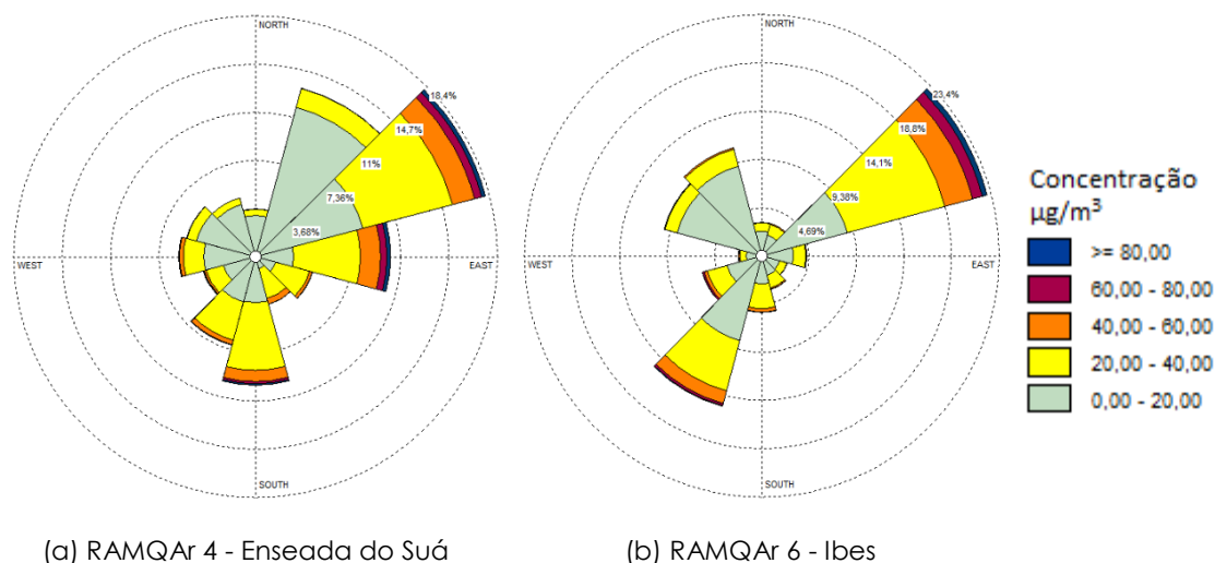
Gráfico 6.7 - Perfil de concentração média de PM 10 nas estações da Enseada do Suá e Ibes.
