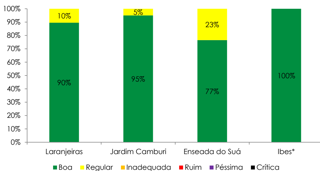
Gráfico 6.23 - Índice de qualidade do ar referente ao poluente NO 2 nas estações da RAMQAr.
