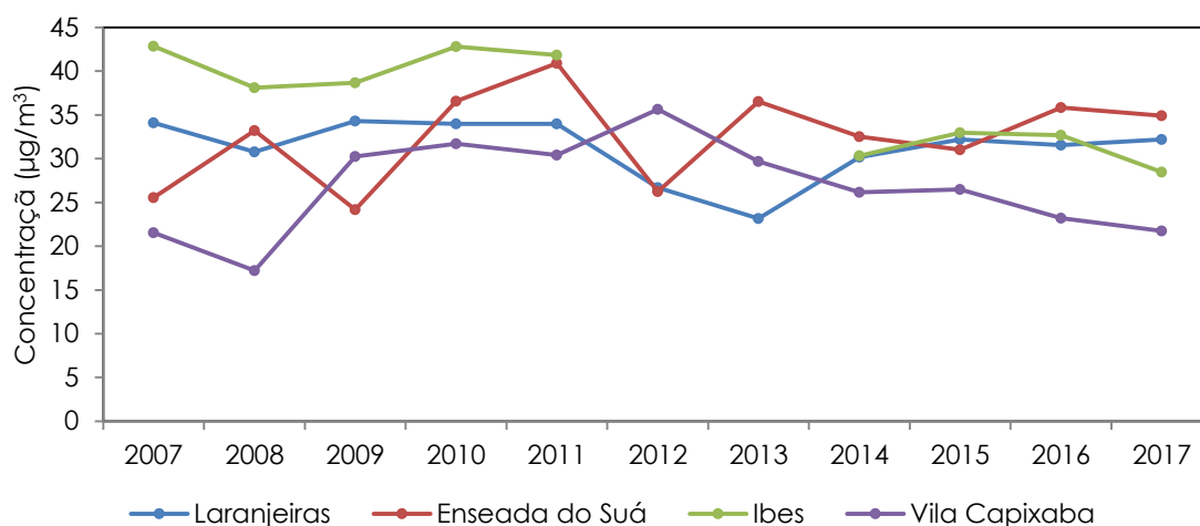
Gráfico 6.31 - Séries temporais das concentrações médias anuais do O 3 nas estações da RAMQAr.
