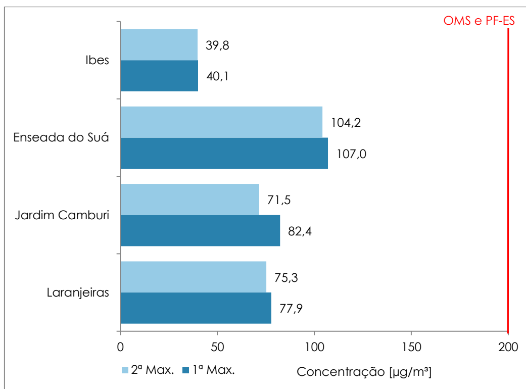
Gráfico 6.21 - Concentrações horária máximas de NO 2 nas estações da RAMQAr.
