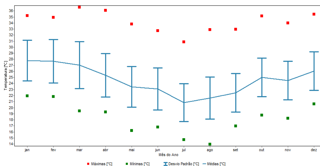
Gráfico 5.2 - Temperatura média mensal, máxima e mínima nas estações da RAMQAr.
