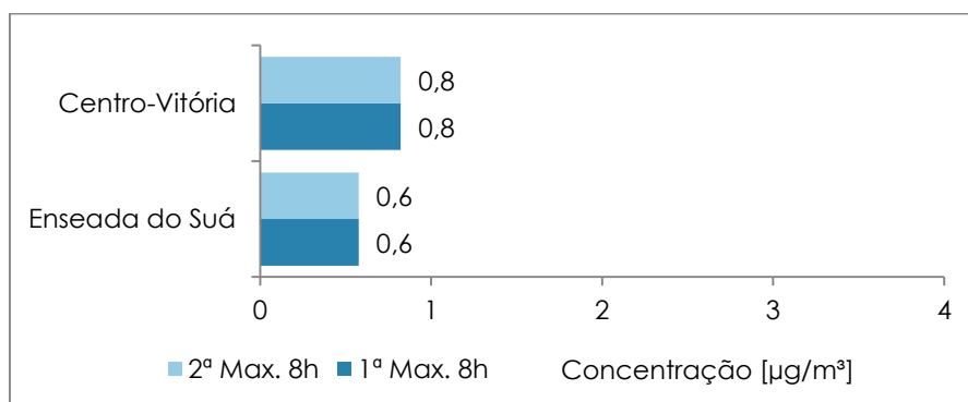
Gráfico 6.37 - Concentração média 8h máxima de HCNM nas estações da RAMQAr.
