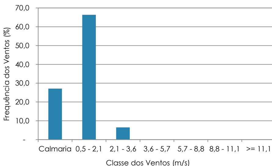
Gráfico 5.9 - Distribuição de frequência de ocorrência das classes de vento nas estações avaliadas da RMGV.
