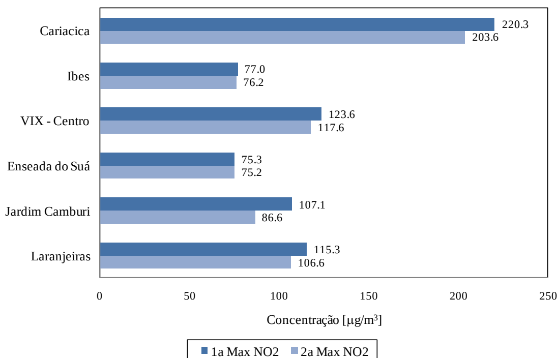
Figura 7.14. Concentrações horárias máximas de \text{NO}_2 nas estações da RAMQAr (ano base 2010). OMS representa a diretriz da Organização Mundial de Saúde para o referido poluente, que equivale ao padrão final preconizado na legislação estadual (PF-ES).
