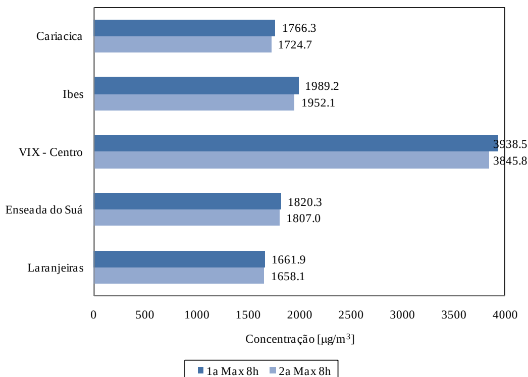
Figura 7.22. Concentração média de 8h máxima de CO nas estações da RAMQAr (ano base 2010).
