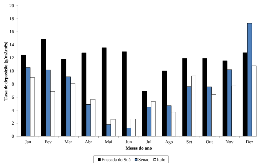
Figura 7.9. Taxa de deposição de partículas ( \text{g/m}^2/30 dias) nas estações de monitoramento de PS (ano base 2010).
