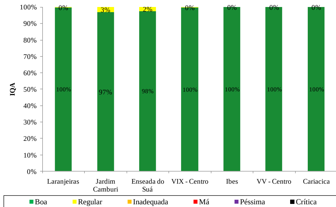
Figura 7.12. Índice de qualidade do ar com referência ao poluente SO 2 nas estações da RAMQAr (ano base 2010).
