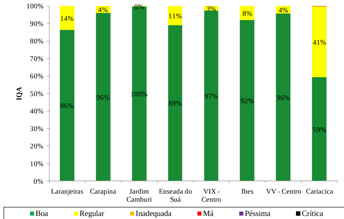
Figura 7.3. Índice de qualidade do ar com referencia ao poluente MP_{10} nas estações da RAMQAr (ano base 2010).
