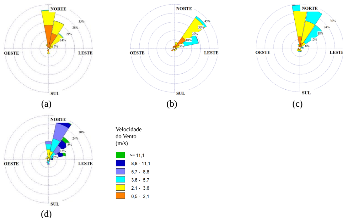
Figura 6.23. Rosa dos ventos para o mês de dezembro nas estações: (a) Carapina; (b) Enseada do Suá; (c) Ibes; e (d) Aeroporto.
