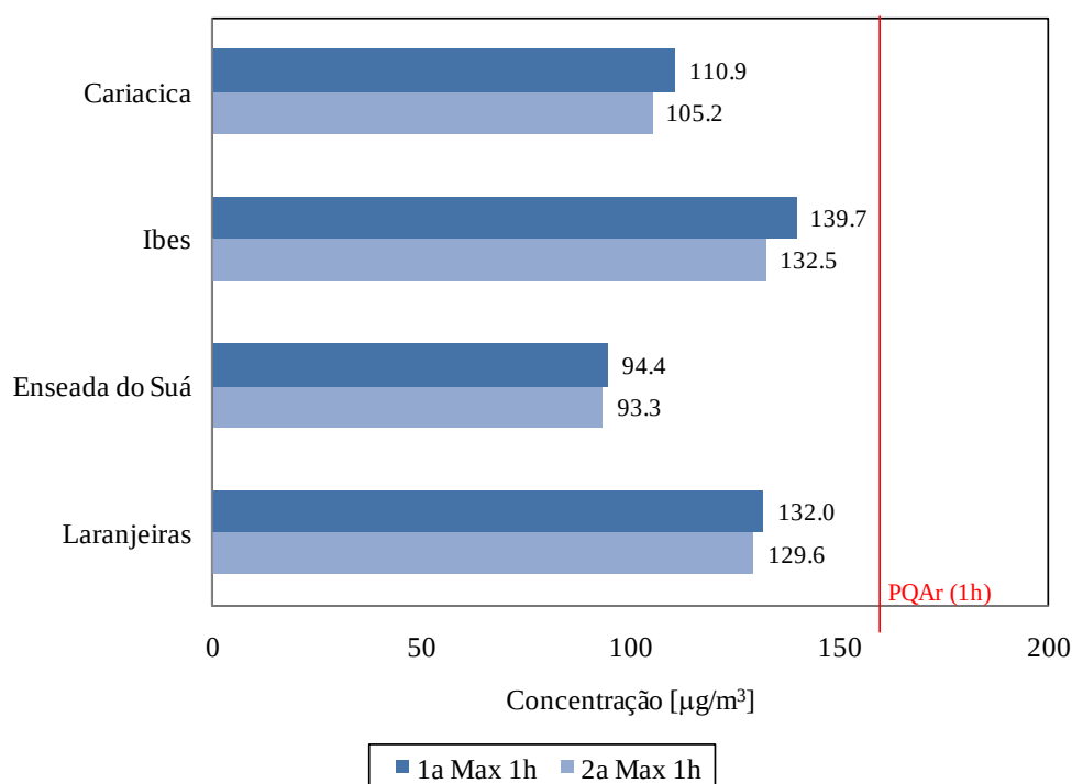
Figura 7.19. Concentração horária máxima de O_3 nas estações da RAMQAr (ano base 2010). PQAr indica o padrão nacional de qualidade do ar. Valores destacados com * são considerados não-representativos.
