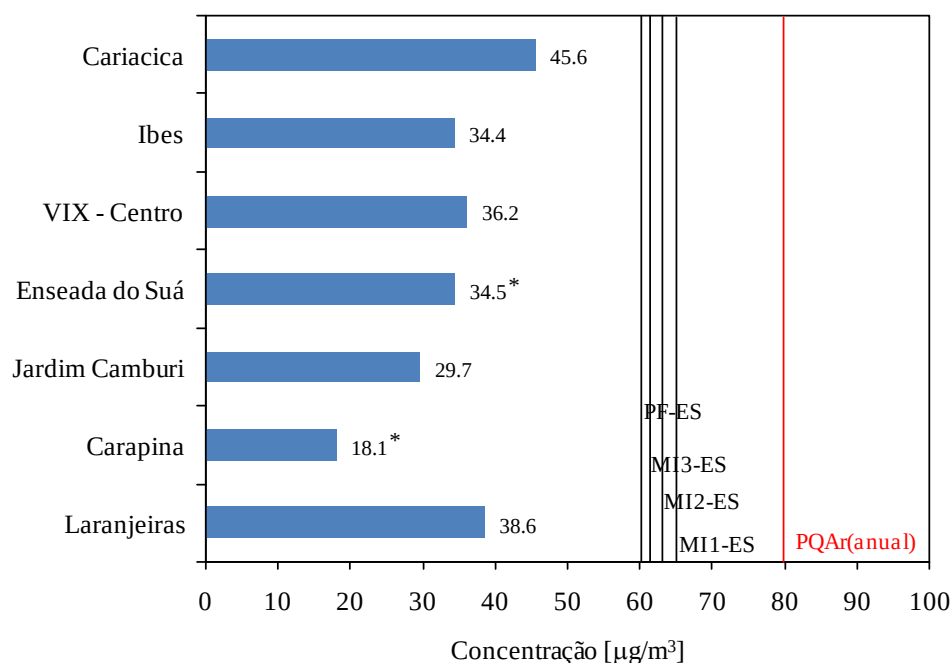
Figura 7.6. Concentração média anual de PTS nas estações da RAMQAr (ano base 2010). PQAr indica o padrão nacional de qualidade do ar. MI1-ES, MI2-ES e MI3-ES são as metas intermediárias e PF-ES é o padrão final preconizado na legislação estadual. Valores destacados com * são considerados não-representativos.
