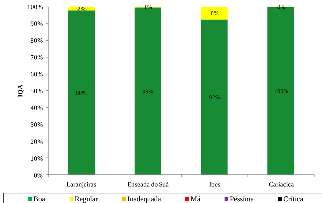
Figura 7.20. Índice de qualidade do ar com referência ao poluente O 3 nas estações da RAMQAr (ano base 2010).
