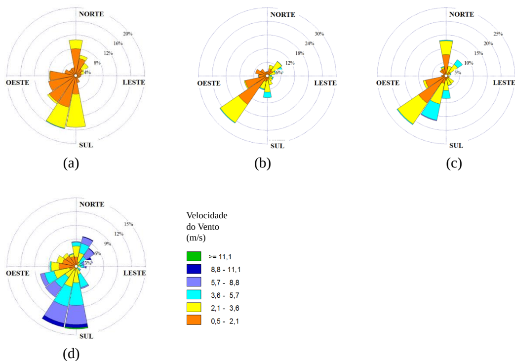
Figura 6.15. Rosa dos ventos para o mês de abril nas estações: (a) Carapina; (b) Enseada do Suá; (c) Ibes; e (d) Aeroporto.
