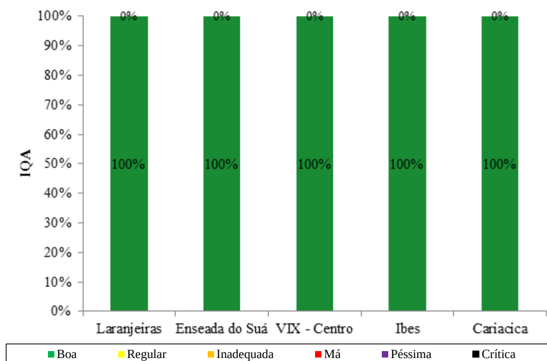
Figura 7.24. Índice de qualidade do ar com referência ao poluente CO nas estações da RAMQAr (ano base 2010).
