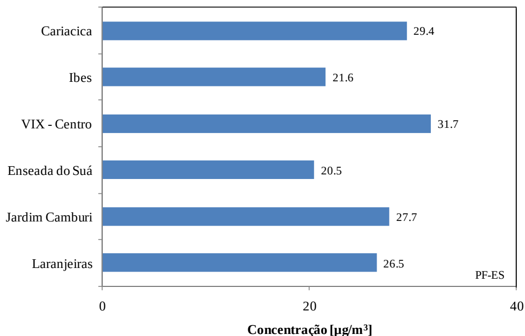
Figura 7.15. Concentrações médias anuais de NO 2 nas estações da RAMQAr (ano base 2010). PF-ES é o padrão final preconizado na legislação estadual.
