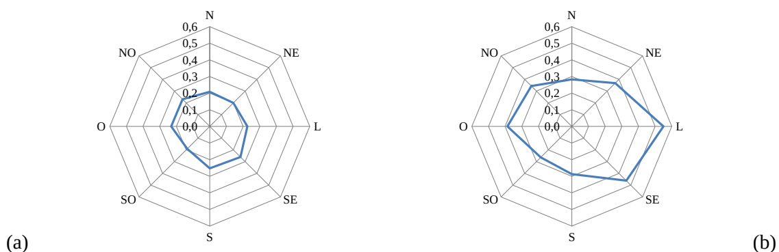
Figura 7.28. Perfil de concentração média horária de HCNM nas estações da RAMQAr com relação à direção do vento (gráfico de radar): (a) Enseada do Suá** e (b) VIX-Centro**. Utilizado os dados de direção do vento da estação SBVT 83649 – Aeroporto de Vitória.
