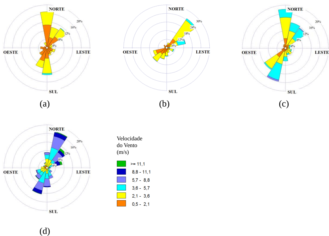
Figura 6.21. Rosa dos ventos para o mês de outubro nas estações: (a) Carapina; (b) Enseada do Suá; (c) Ibes; e (d) Aeroporto.
