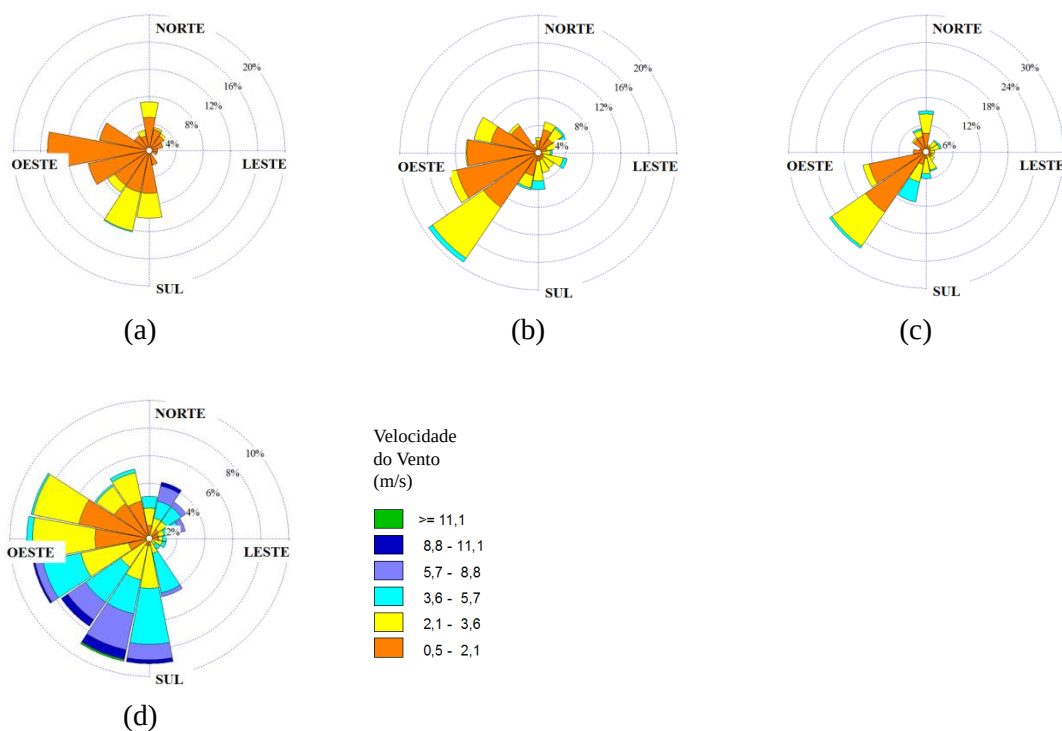
Figura 6.17. Rosa dos ventos para o mês de junho nas estações: (a) Carapina; (b) Enseada do Suá; (c) Ibes; e (d) Aeroporto.
