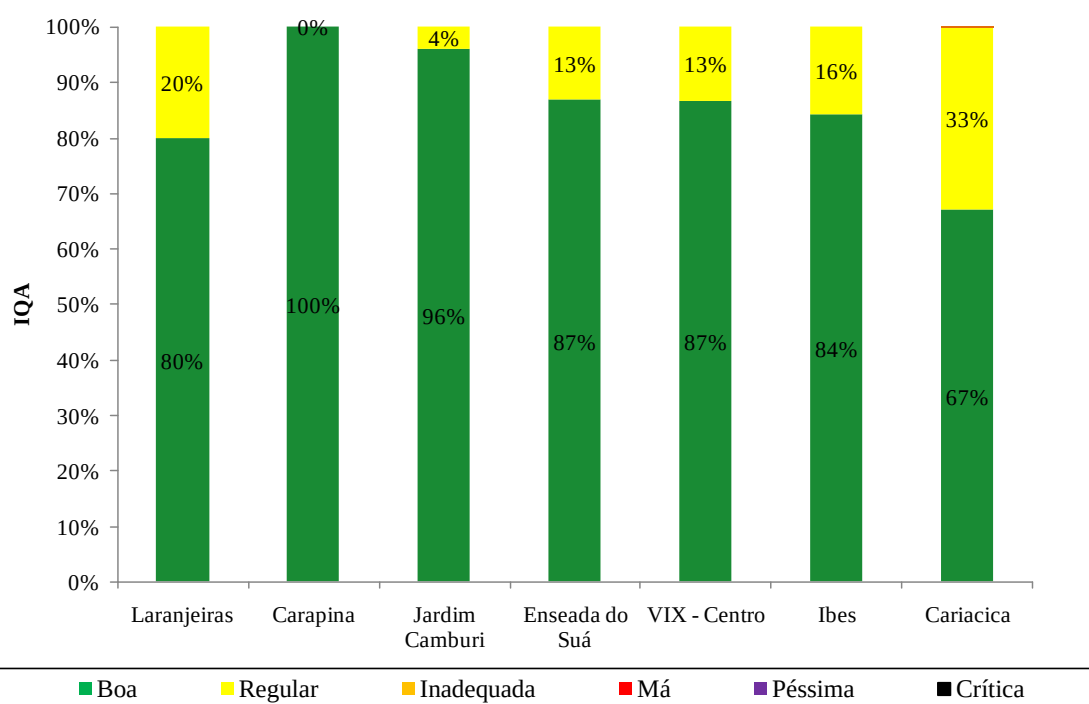
Figura 7.7. Índice de qualidade do ar com base no poluente PTS nas estações da RAMQAr (ano base 2010).
