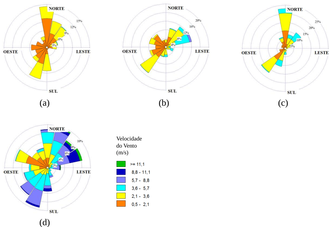
Figura 6.19. Rosa dos ventos para o mês de agosto nas estações: (a) Carapina; (b) Enseada do Suá; (c) Ibés; e (d) Aeroporto.
