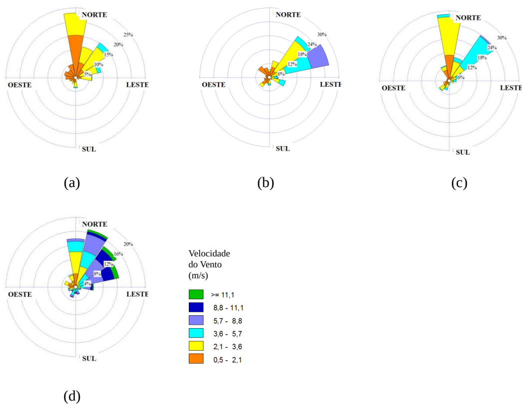
Figura 6.13. Rosa dos ventos para o mês de fevereiro nas estações: (a) Carapina; (b) Enseada do Suá; (c) Ibes; e (d) Aeroporto.
