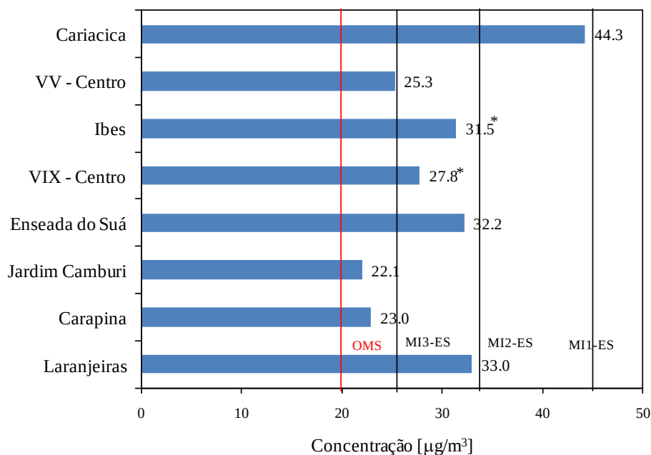
Figura 7.2. Concentração média anual de MP 10 nas estações da RAMQAr (ano base 2010). PQAr indica o padrão nacional de qualidade do ar. MI1-ES, MI2-ES e MI3-ES são as metas intermediárias. OMS representa a diretriz da Organização Mundial de Saúde para o referido poluente, que equivale ao padrão final preconizado na legislação estadual (PF-ES). Valores destacados com * são considerados não-representativos.
