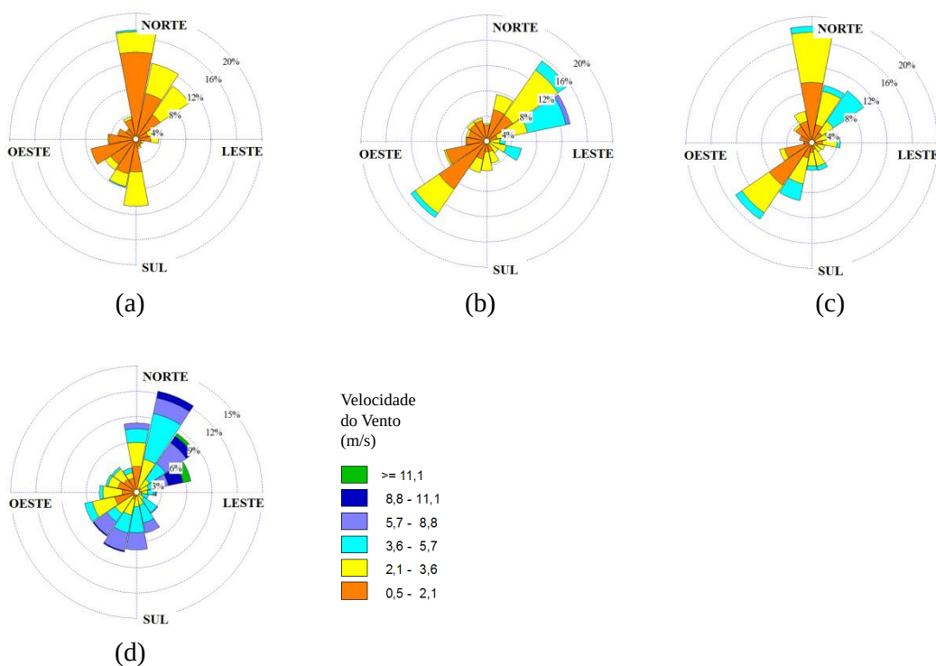
Figura 6.14. Rosa dos ventos para o mês de março nas estações: (a) Carapina; (b) Enseada do Suá; (c) Ibes; e (d) Aeroporto.
