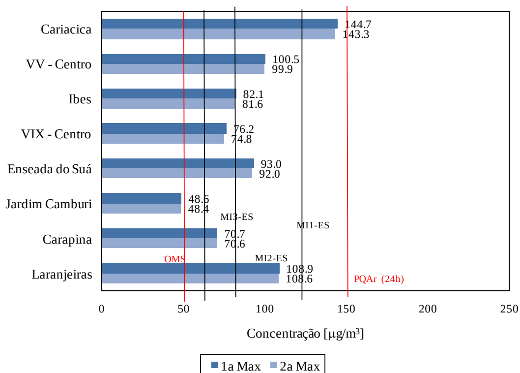
Figura 7.1. Concentração máxima média de 24h de MP_{10} nas estações da RAMQAr (ano base 2010). PQAr indica o padrão nacional de qualidade do ar. MI1-ES, MI2-ES e MI3-ES são as metas intermediárias. OMS representa a diretriz da Organização Mundial de Saúde para o referido poluente, que equivale ao padrão final preconizado na legislação estadual (PF-ES). Valores destacados com * são considerados não-representativos.
