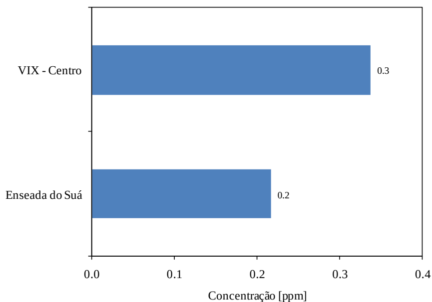
Figura 7.27. Concentração média anual de HCNM nas estações da RAMQAr (ano base 2010).
