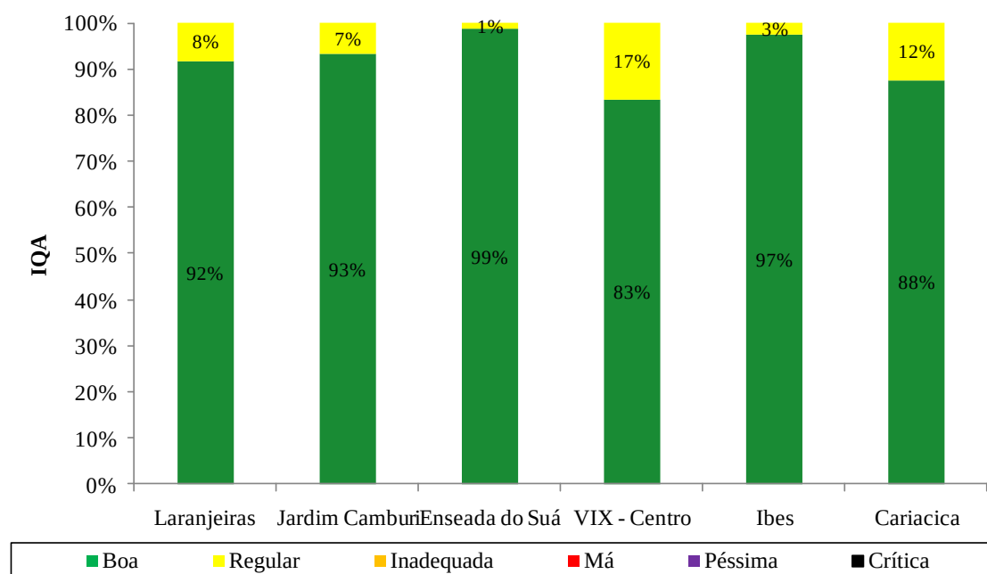
Figura 7.16. Índice de qualidade do ar referente ao poluente NO 2 nas estações da RAMQAr (ano base 2010).
