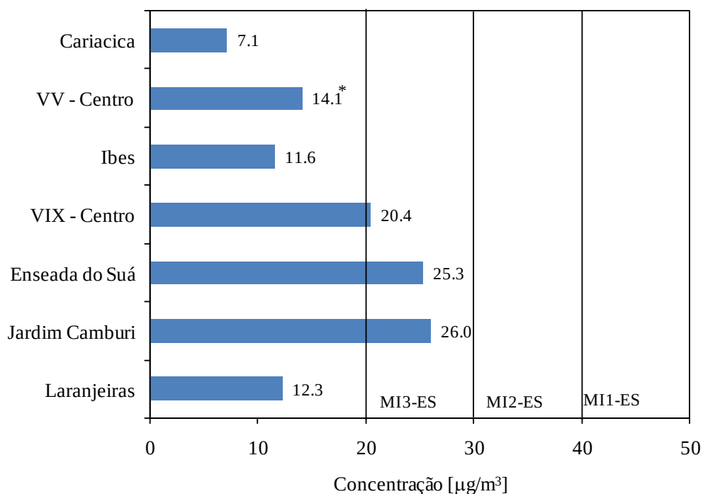
Figura 7.11. Concentração média anual de SO 2 nas estações da RAMQAr (ano base 2010). PQAr indica o padrão nacional de qualidade do ar. MI1-ES, MI2-ES e MI3-ES são as metas intermediárias. Valores destacados com * são considerados não-representativos.
