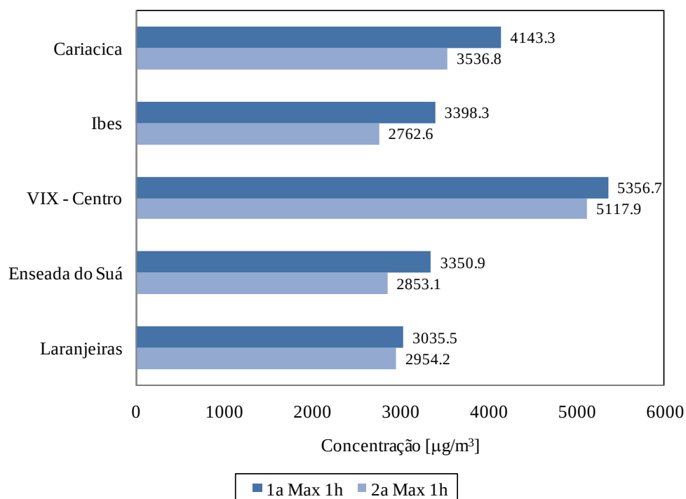
Figura 7.23. Concentração horária máxima de CO nas estações da RAMQAr (ano base 2010).
