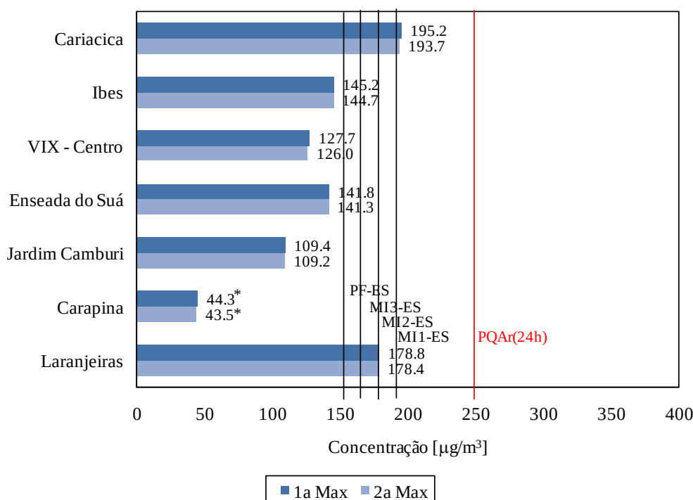
Figura 7.5. Concentração máxima média de 24h de PTS nas estações da RAMQAr (ano base 2010). PQAr indica o padrão nacional de qualidade do ar. MI1-ES, MI2-ES e MI3-ES são as metas intermediárias e PF-ES é o padrão final preconizado na legislação estadual. Valores destacados com * são considerados não-representativos.
