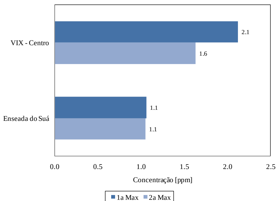
Figura 7.26. Concentração diária máxima de HCNM nas estações da RAMQAr (ano base 2010).
