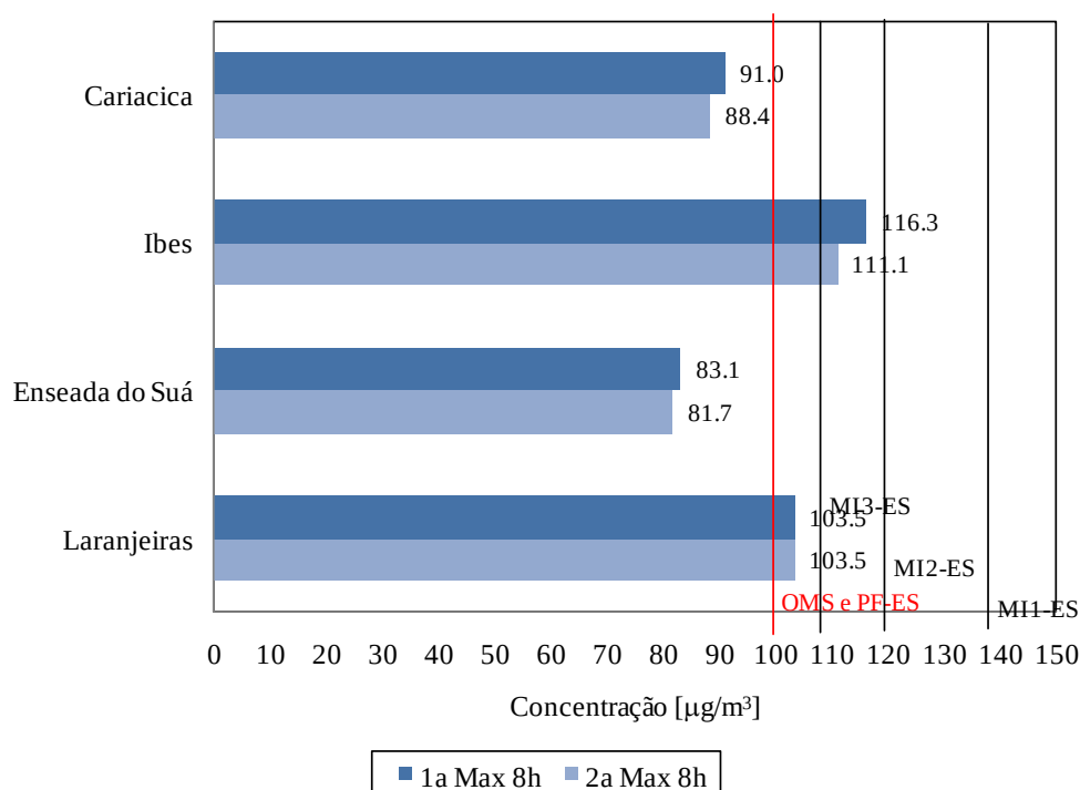
Figura 7.18. Concentração média 8h máxima de O 3 nas estações da RAMQAr (ano base 2010). PQAr indica o padrão nacional de qualidade do ar. MI1-ES, MI2-ES e MI3-ES são as metas intermediárias. OMS representa a diretriz da Organização Mundial de Saúde para o referido poluente, que equivale ao padrão final preconizado na legislação estadual (PF-ES). Valores destacados com * são considerados não-representativos.
