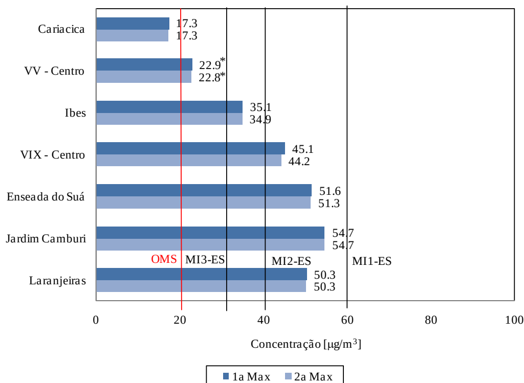
Figura 7.10. Concentração diária máxima de \text{SO}_2 nas estações da RAMQAr (ano base 2010). PQAr indica o padrão nacional de qualidade do ar. MI1-ES, MI2-ES e MI3-ES são as metas intermediárias. OMS representa a diretriz da Organização Mundial de Saúde para o referido poluente, que equivale ao padrão final preconizado na legislação estadual (PF-ES). Valores destacados com * são considerados não-representativos.
