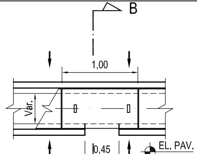
DETALHE CANALETA COM TAMPA DE CONCRETO E ABERTURAS
