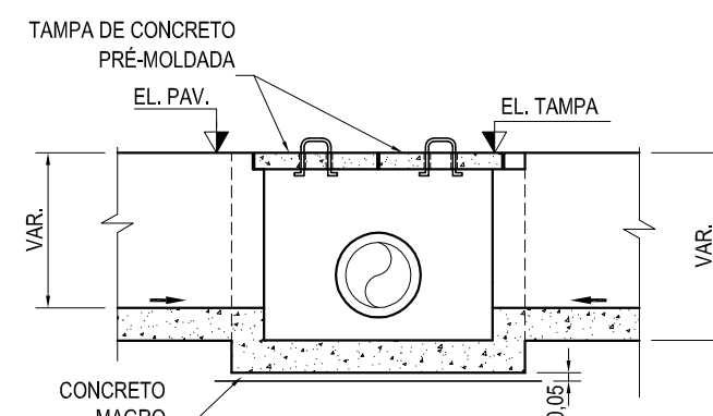
CORTE EE
