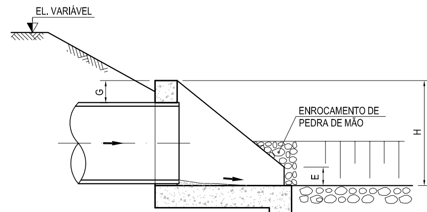
CORTE FF
