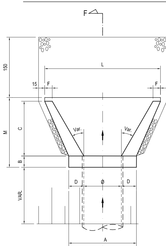
DETALHE TÍPICO DA SAÍDA DE BUEIRO
