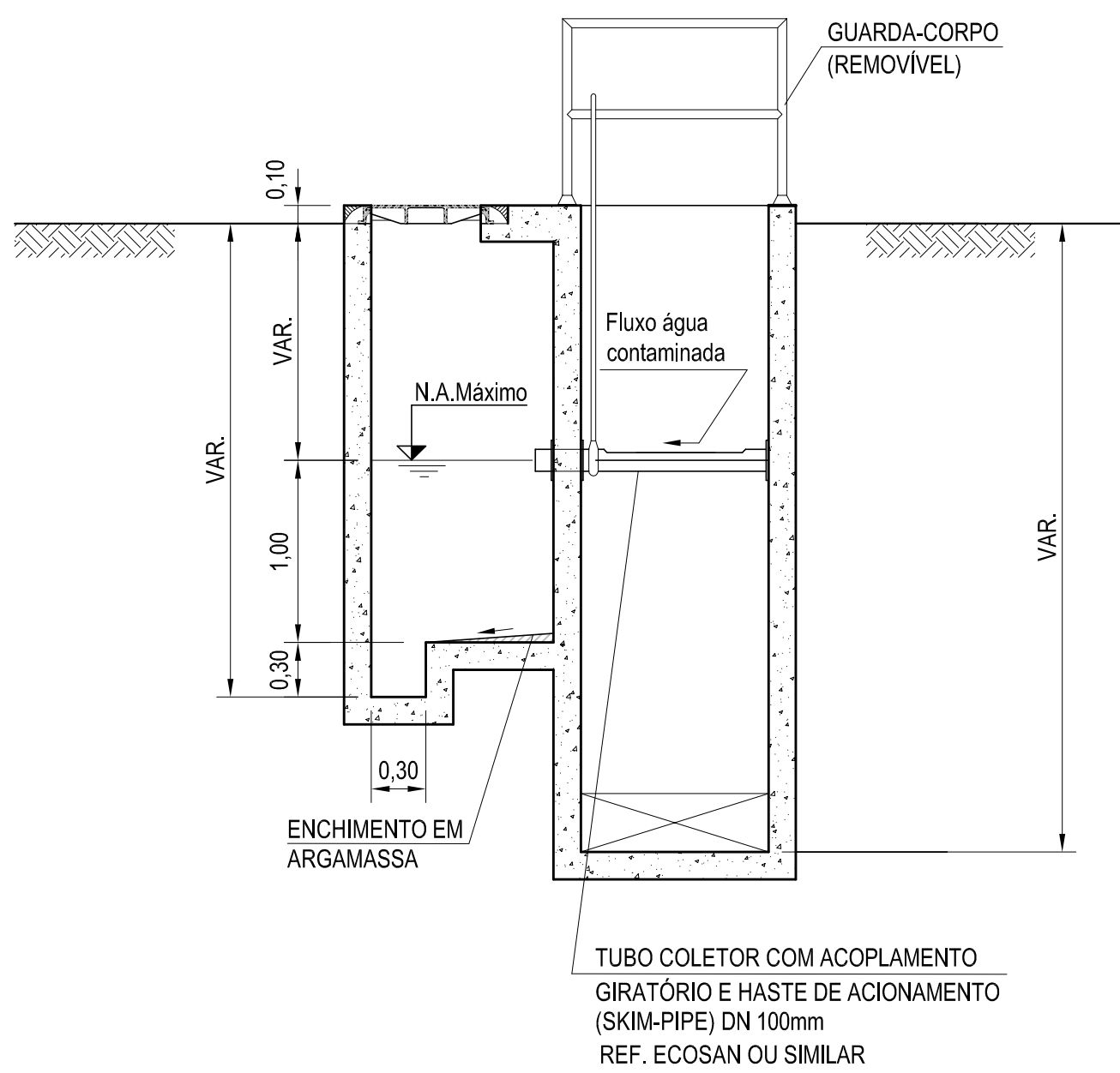
CORTE BB ESC.: 1/150
