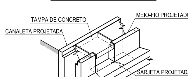
ABERTURA NO MEIO-FIO
