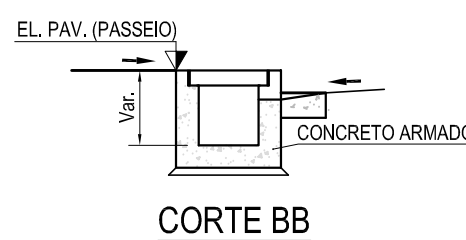
CORTE BB
