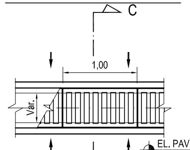
DETALHE CANALETA COM GRELHA DE CONCRETO
