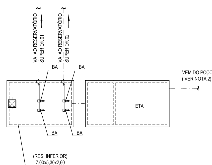
DETALHE 1 - ETA E RESERVATÓRIO INFERIOR DE ÁGUA POTÁVEL S/ESCALA
