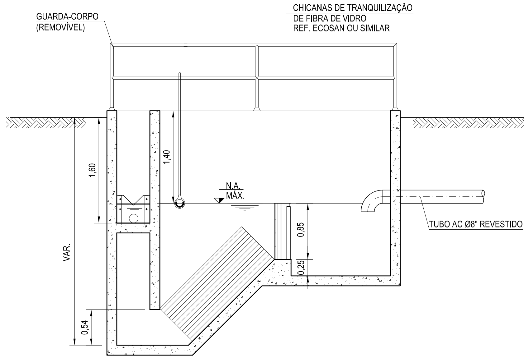
CORTE AA ESC.: 1/150
