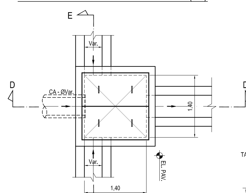
PLANTA
