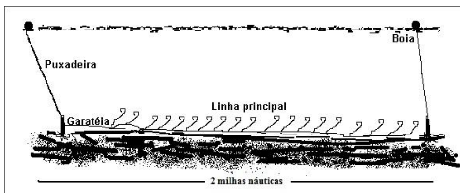
Figura 5.4.9.8.1-5: Desenho esquemático do espinhel de fundo na área de pesca e do equipamento utilizado (Fonte: Furtado Neto et al., 2006, com adaptações)
