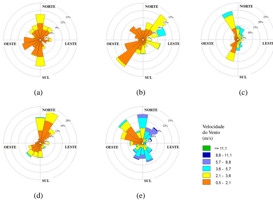
Figura 6.15. Rosa dos ventos para o mês de abril nas estações: (a) Carapina; (b) Enseada do Suá; (c) Ibes; (d) Cariacica; e (e) Aeroporto.
