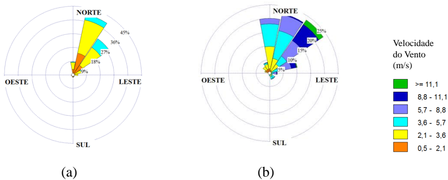
Figura 6.23. Rosa dos ventos para o mês de dezembro nas estações: (a) Cariacica e (b) Aeroporto.
