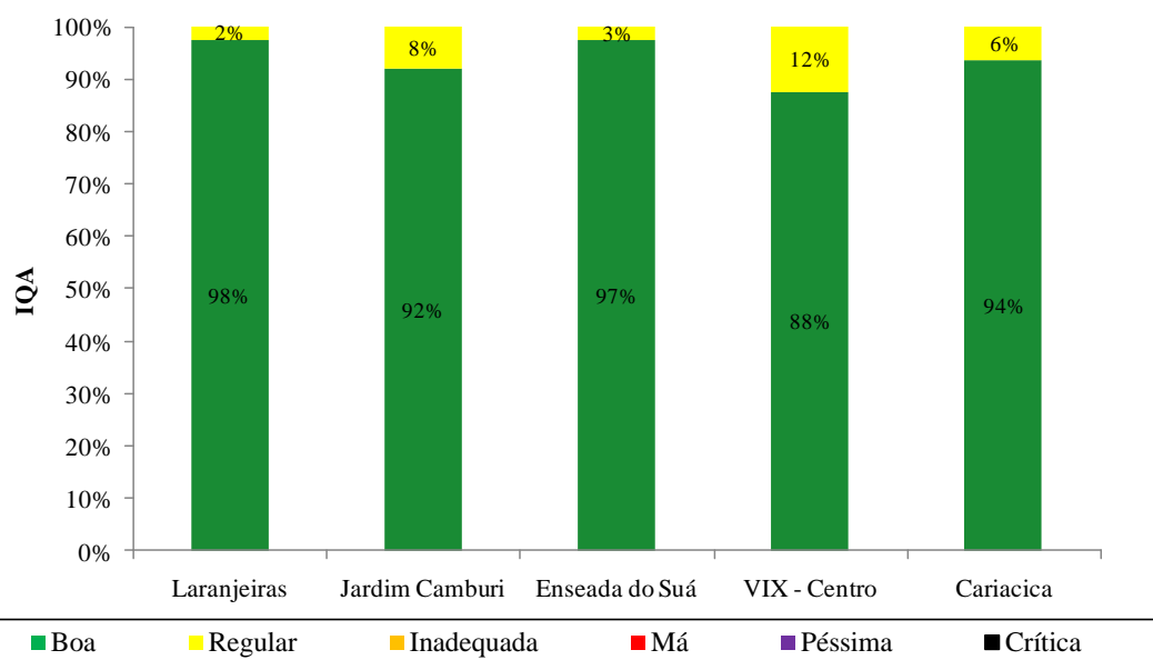
Figura 7.16. Índice de qualidade do ar referente ao poluente NO 2 nas estações da RAMQAr (ano base 2012).
