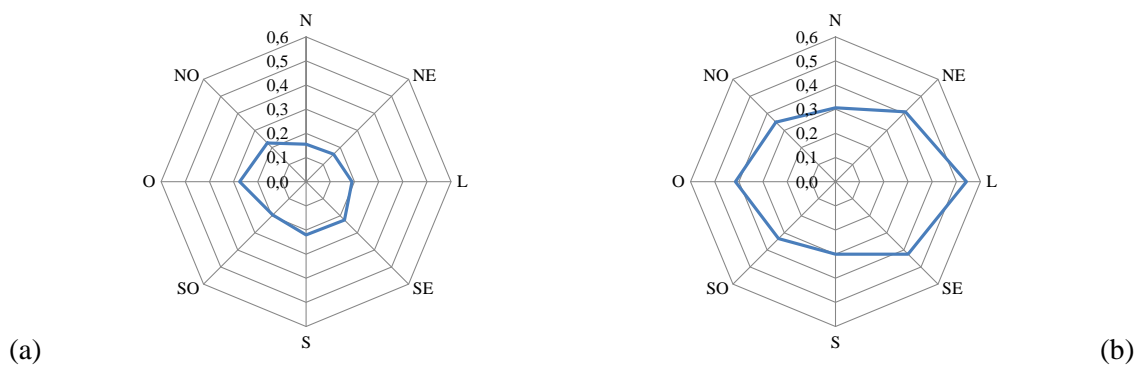
Figura 7.28. Perfil de concentração média horária de HCNM nas estações da RAMQAr com relação à direção do vento (gráfico de radar): (a) Enseada do Suá** e (b) VIX-Centro**.
