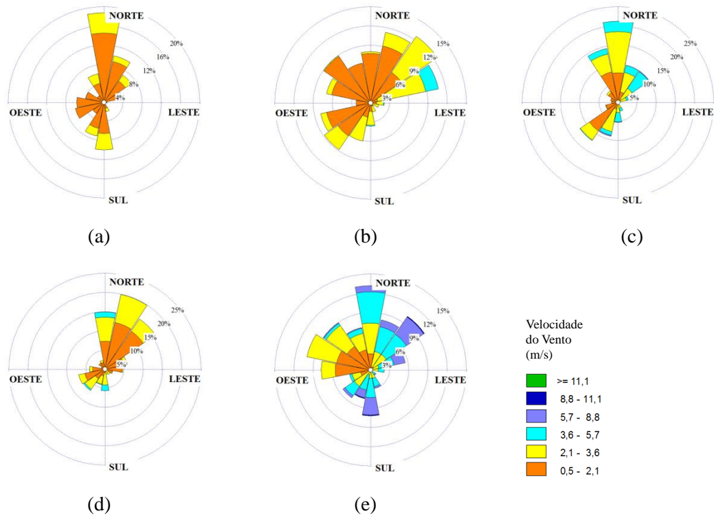
Figura 6.18. Rosa dos ventos para o mês de julho nas estações: (a) Carapina; (b) Enseada do Suá; (c) Ibes; (d) Cariacica; e (e) Aeroporto.
