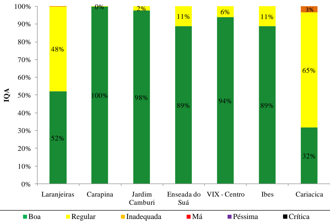
Figura 7.7. Índice de qualidade do ar com referência ao poluente PTS nas estações da RAMQAr (ano base 2012).
