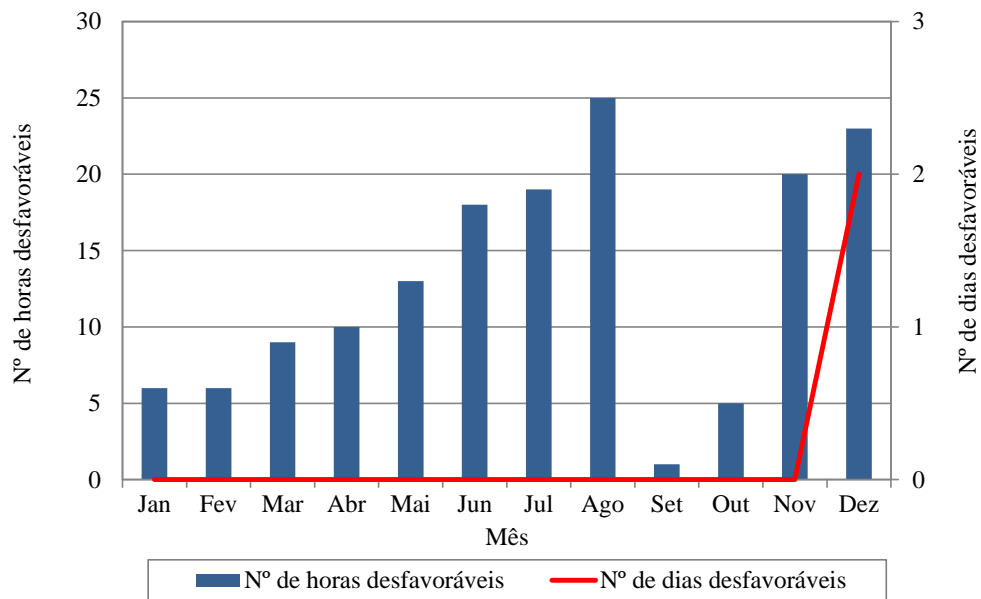
Figura 6.24. Número de horas e dias desfavoráveis à dispersão de poluentes.
