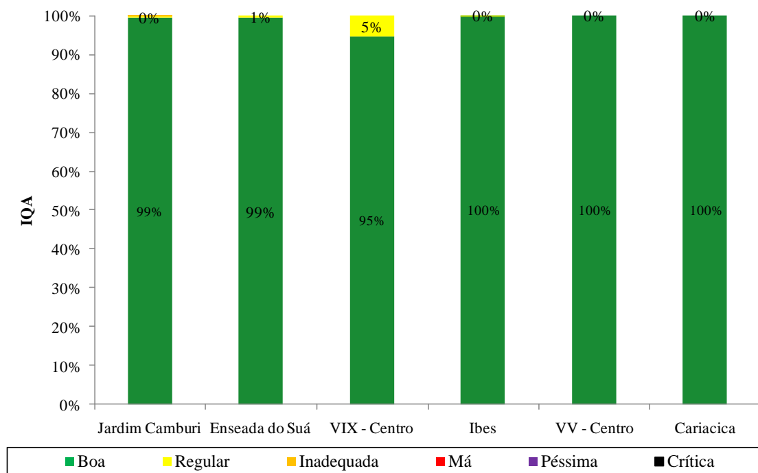
Figura 7.12. Índice de qualidade do ar com referência ao poluente \text{SO}_2 nas estações da RAMQAr (ano base 2012).
