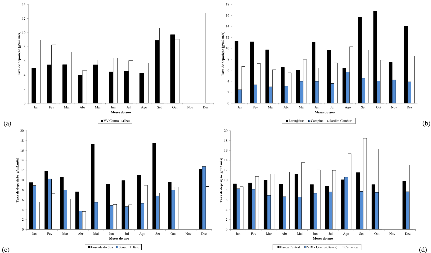
Figura 7.9. Taxa de deposição de partículas ( \text{g}/\text{m}^2/30 dias) nas estações de monitoramento de PS (ano base 2012).
