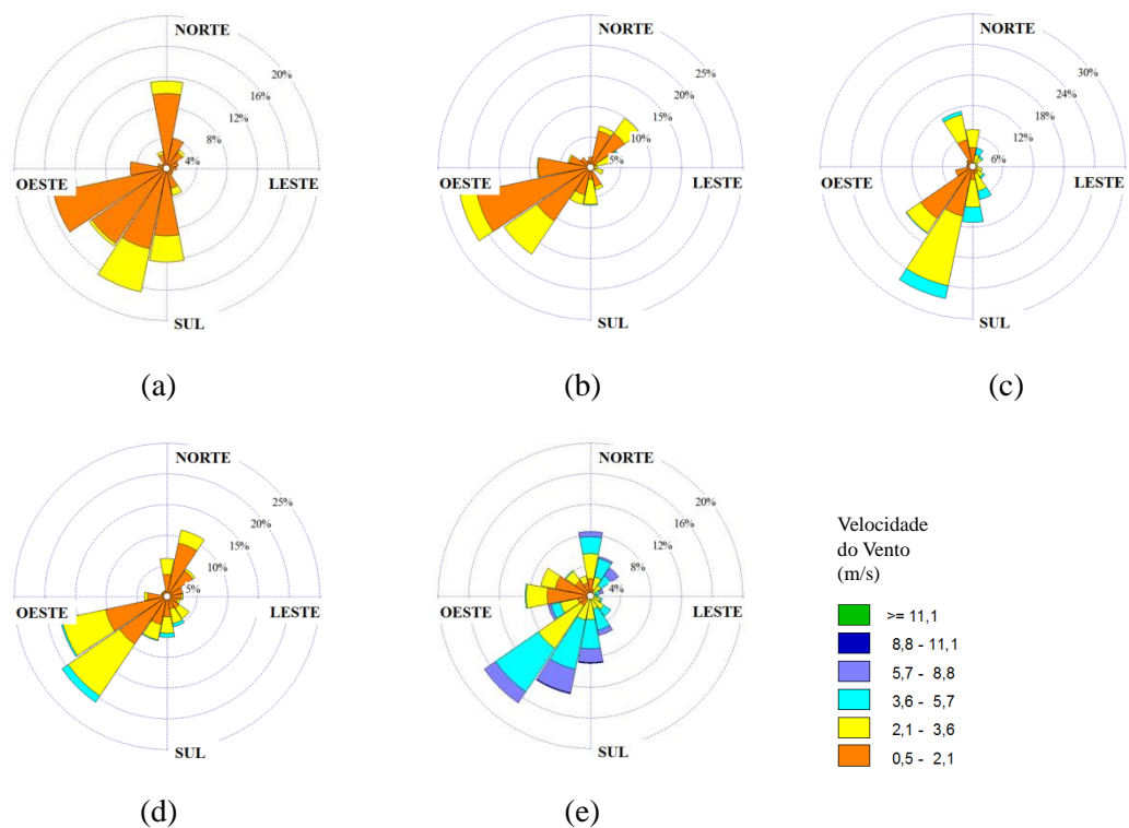
Figura 6.16. Rosa dos ventos para o mês de maio nas estações: (a) Carapina; (b) Enseada do Suá; (c) Ibes; (d) Cariacica; e (e) Aeroporto.
