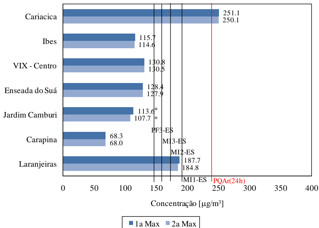
Figura 7.5. Concentração máxima média de 24h de PTS nas estações da RAMQAr (ano base 2012). PQAr indica o padrão nacional de qualidade do ar. MI1-ES, MI2-ES e MI3-ES são as metas intermediárias e PF-ES é o padrão final preconizado na legislação estadual. Valores destacados com * são considerados não-representativos.
