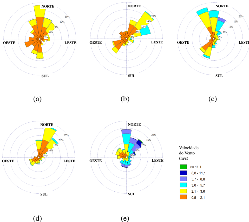
Figura 6.10. Rosa dos ventos anual nas estações: (a) Carapina; (b) Enseada do Suá; (c) Ibes; (d) Cariacica; e (e) Aeroporto.
