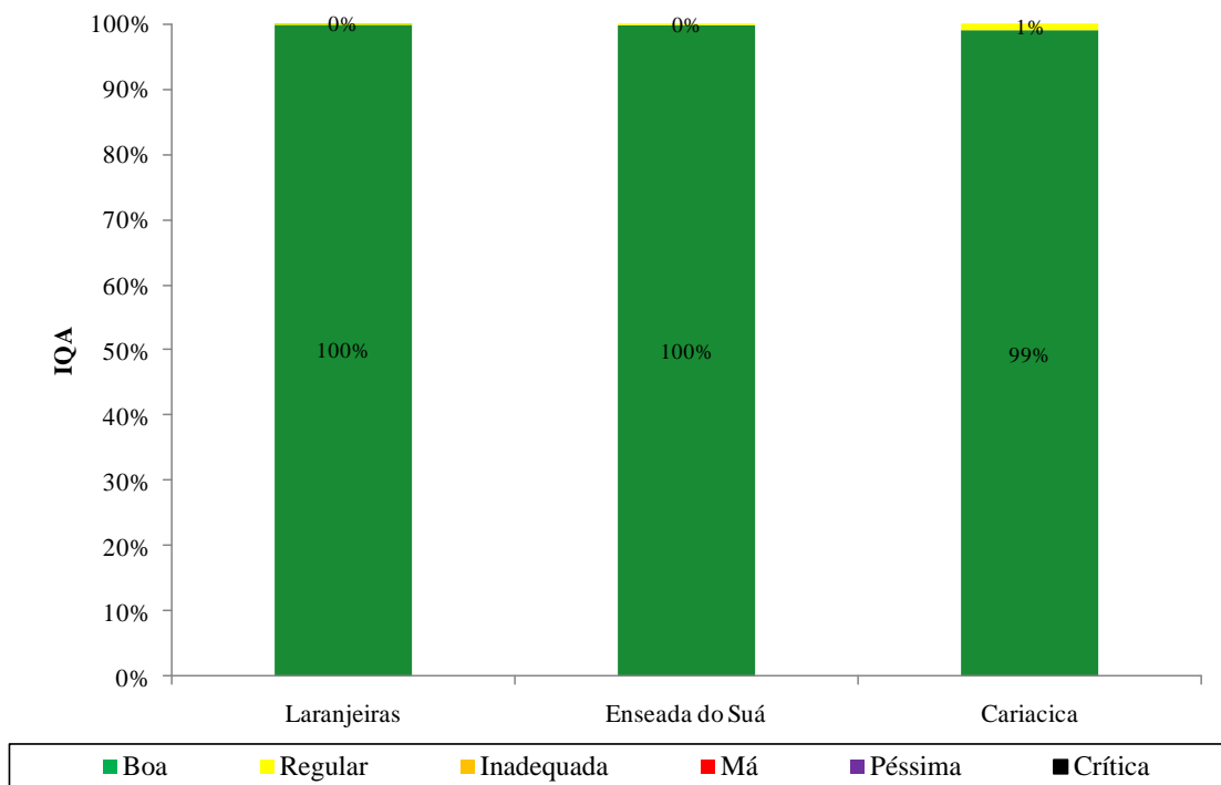
Figura 7.20. Índice de qualidade do ar com referência ao poluente O 3 nas estações da RAMQAr (ano base 2012).
