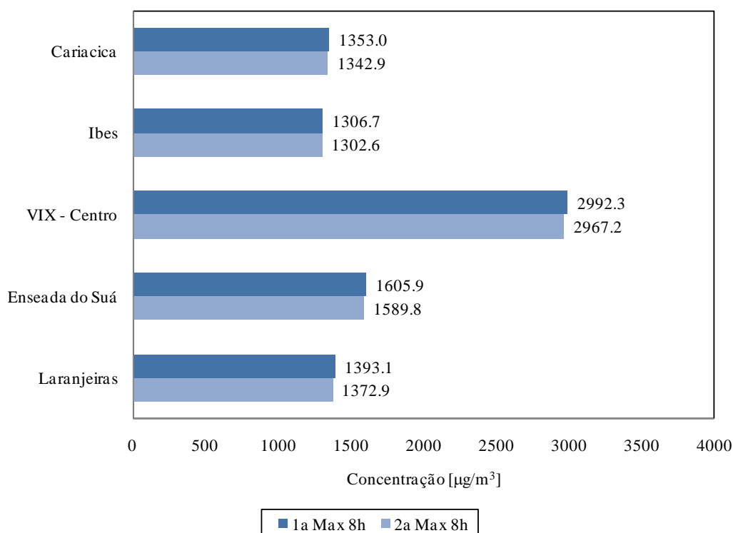
Figura 7.22. Concentração média de 8h máxima de CO nas estações da RAMQAr (ano base 2012).
