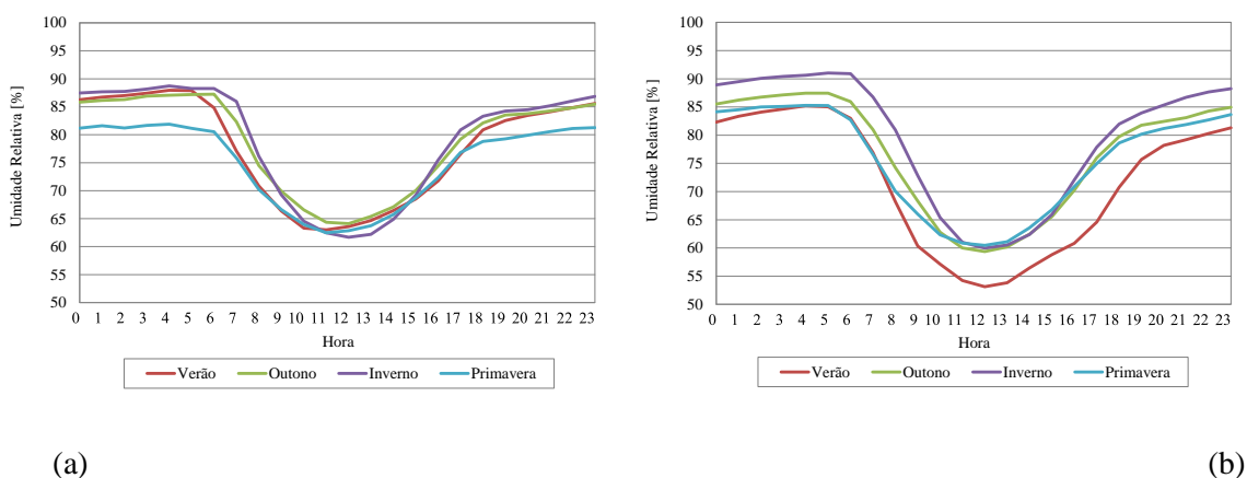
Figura 6.7. Umidade relativa média horária nos períodos de solstício e equinócio nas estações: (a) Carapina e (b) Cariacica.
