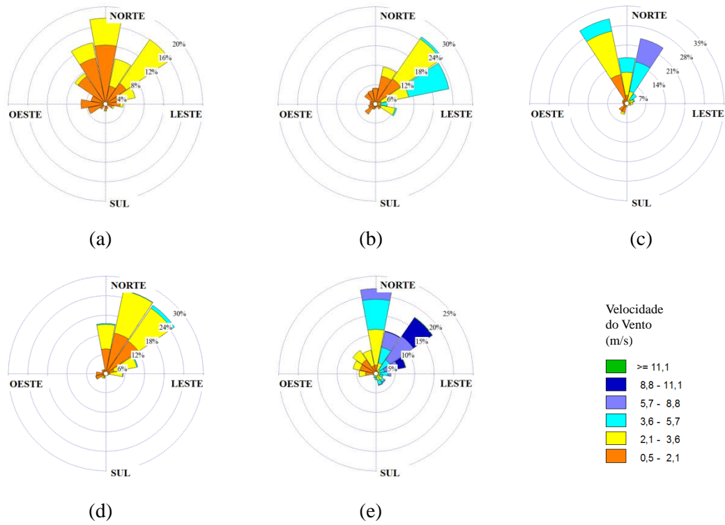
Figura 6.13. Rosa dos ventos para o mês de fevereiro nas estações: (a) Carapina; (b) Enseada do Suá; (c) Ibes; (d) Cariacica; e (e) Aeroporto.
