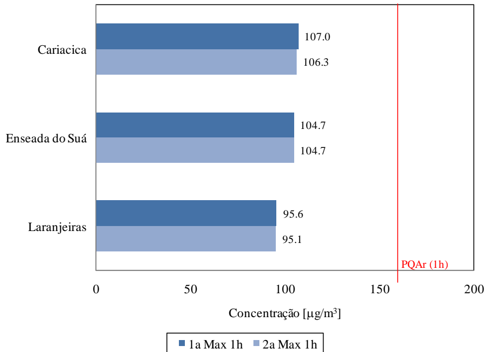
Figura 7.19. Concentração horária máxima de O 3 nas estações da RAMQAr (ano base 2012). PQAr indica o padrão nacional de qualidade do ar. Valores destacados com * são considerados não-representativos.
