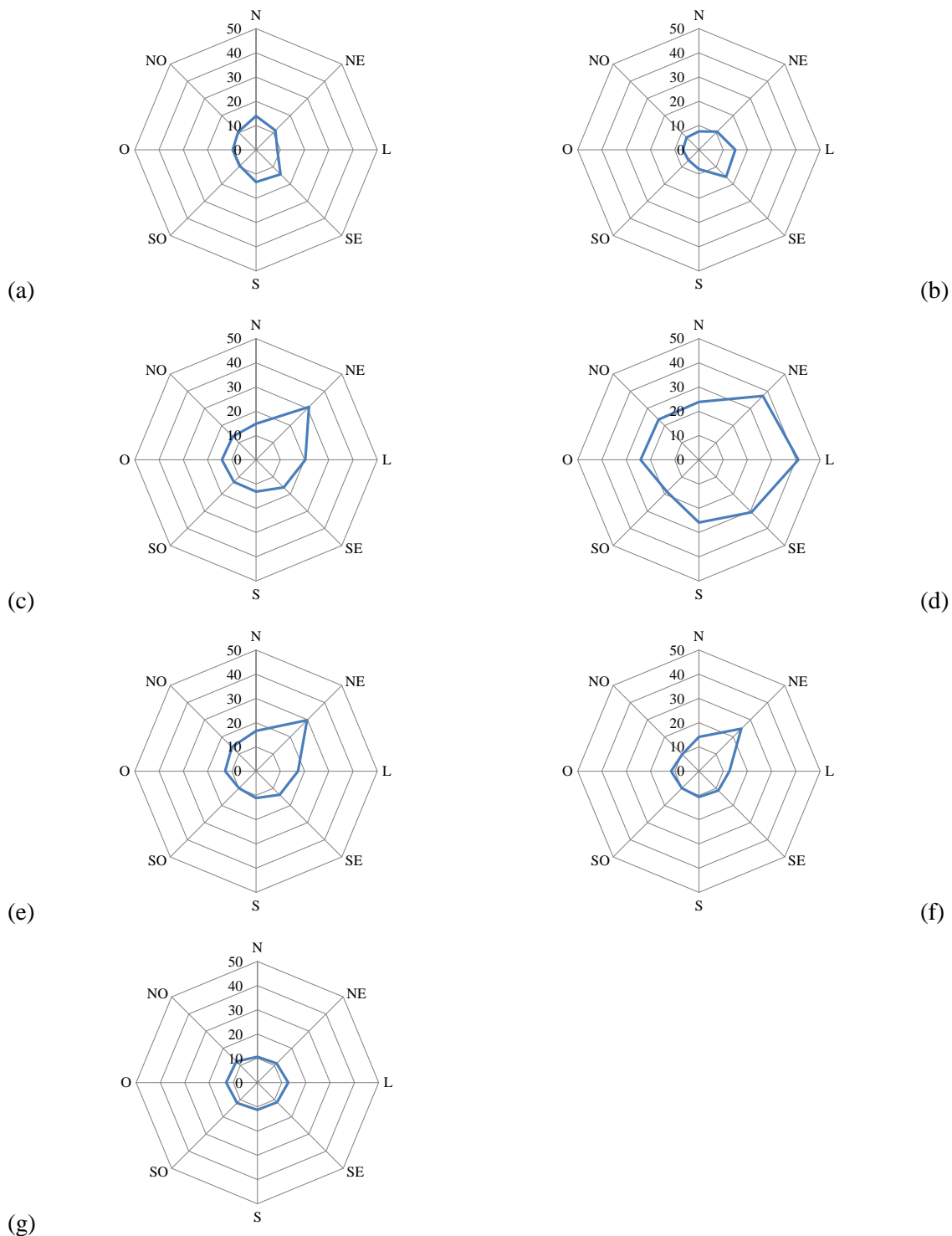
Figura 7.13. Perfil de concentração média horária de \text{SO}_2 nas estações da RAMQAr com relação à direção do vento** (gráfico de radar): (a) Laranjeiras; (b) Jardim Camburi; (c) Enseada do Suá; (d) VIX-Centro; (e) Ibes; (f) VV-Centro e (g) Cariacica.
