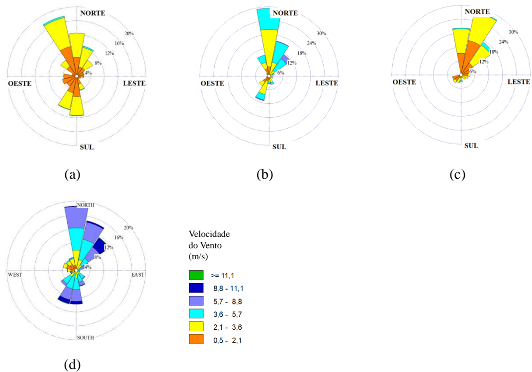
Figura 6.20. Rosa dos ventos para o mês de setembro nas Estações: (a) Carapina; (b) Ibes; (c) Cariacica; e (d) Aeroporto.
