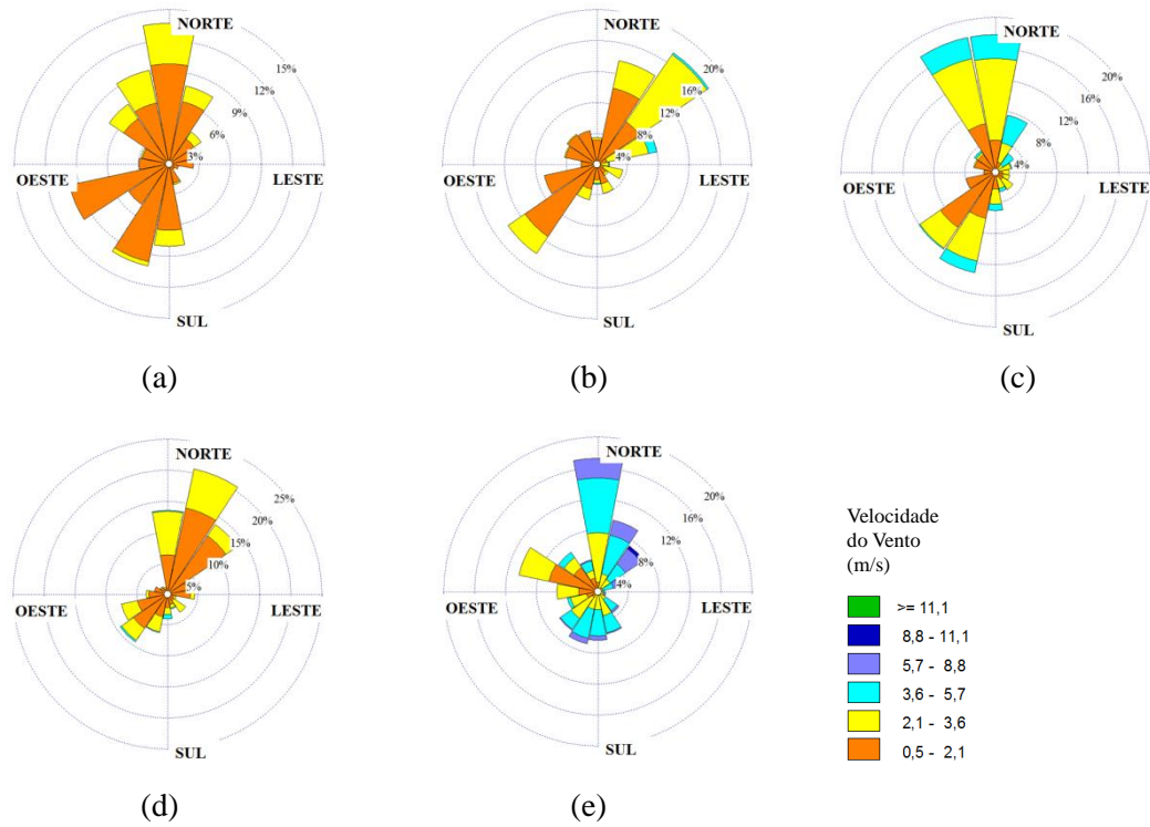
Figura 6.17. Rosa dos ventos para o mês de junho nas estações: (a) Carapina; (b) Enseada do Suá; (c) Ibes; (d) Cariacica; e (e) Aeroporto.
