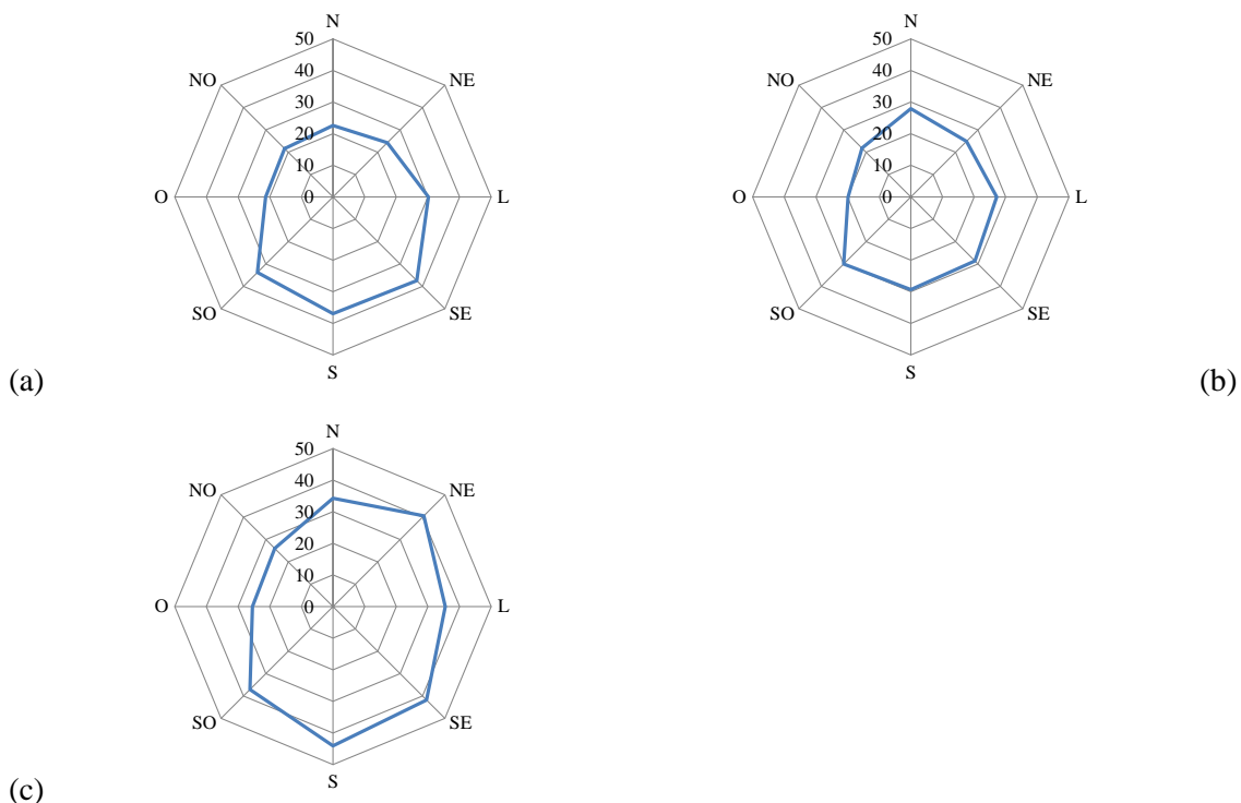
Figura 7.21. Perfil de concentração média horária de O 3 nas estações da RAMQAr com relação à direção do vento (gráfico de radar): (a) Laranjeiras**, (b) Enseada do Suá** e (c) Cariacica**.
