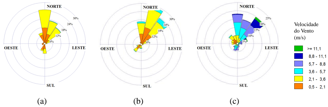
Figura 6.21. Rosa dos ventos para o mês de outubro nas estações: (a) Carapina, (b) Cariacica e (c) Aeroporto.
