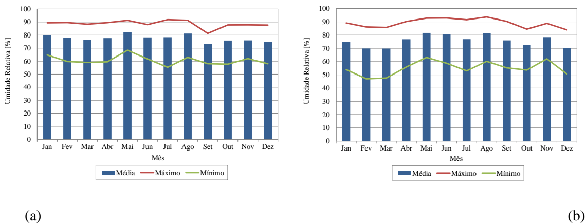
Figura 6.8. Umidade relativa média mensal, máxima e mínima nas estações: (a) Carapina e (b) Cariacica.
