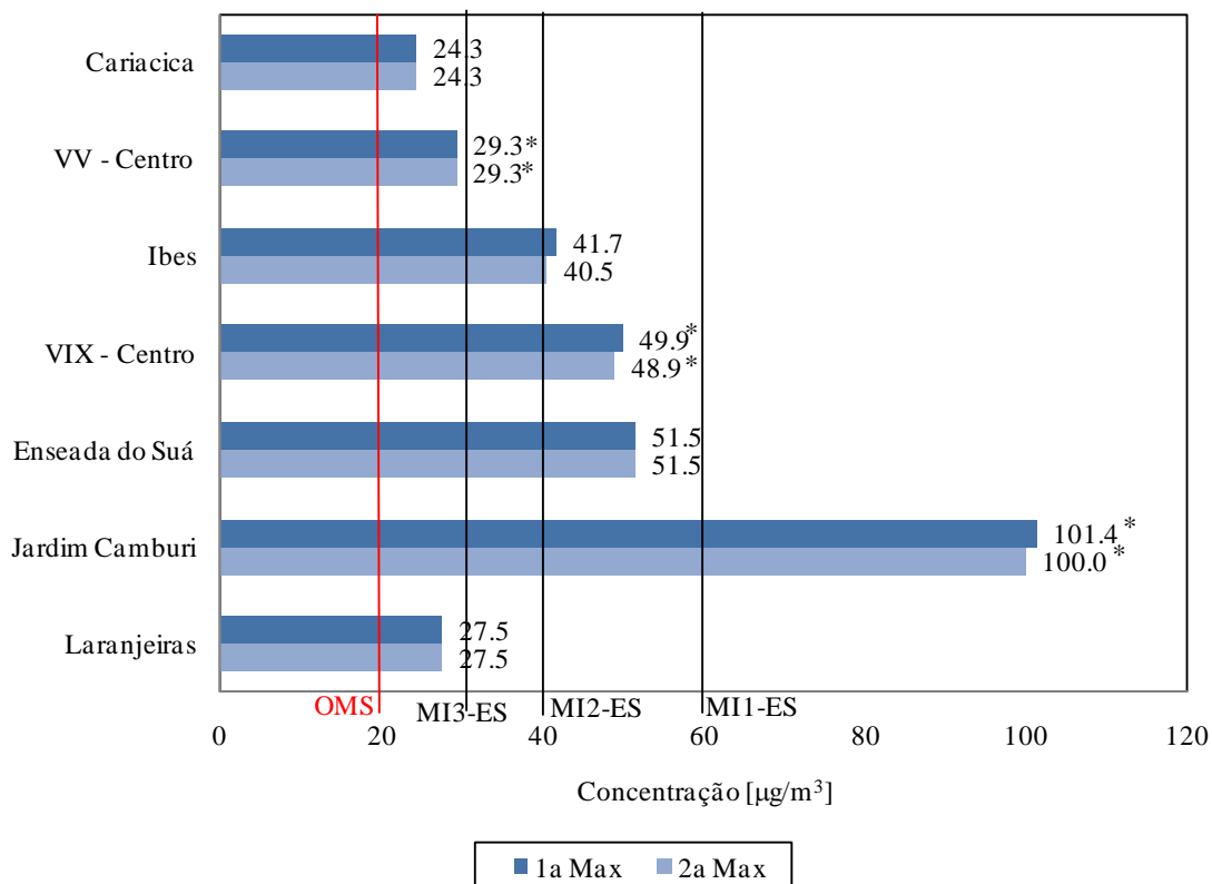
Figura 7.10. Concentração diária máxima de SO 2 nas estações da RAMQAr (ano base 2012). PQAr indica o padrão nacional de qualidade do ar. MI1-ES, MI2-ES e MI3-ES são as metas intermediárias. OMS representa a diretriz da Organização Mundial de Saúde para o referido poluente, que equivale ao padrão final preconizado na legislação estadual (PF-ES). Valores destacados com * são considerados não-representativos.
