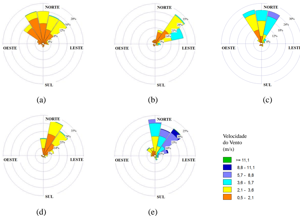
Figura 6.12. Rosa dos ventos para o mês de janeiro nas estações: (a) Carapina; (b) Enseada do Suá; (c) Ibes; (d) Cariacica; e (e) Aeroporto.
