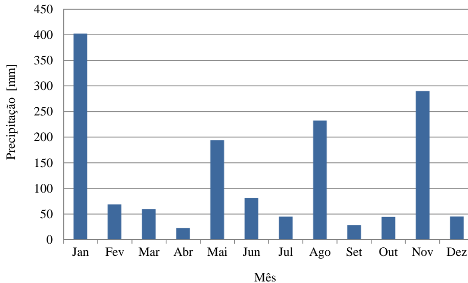
Figura 6.1. Precipitação acumulada mensal na estação Carapina.
