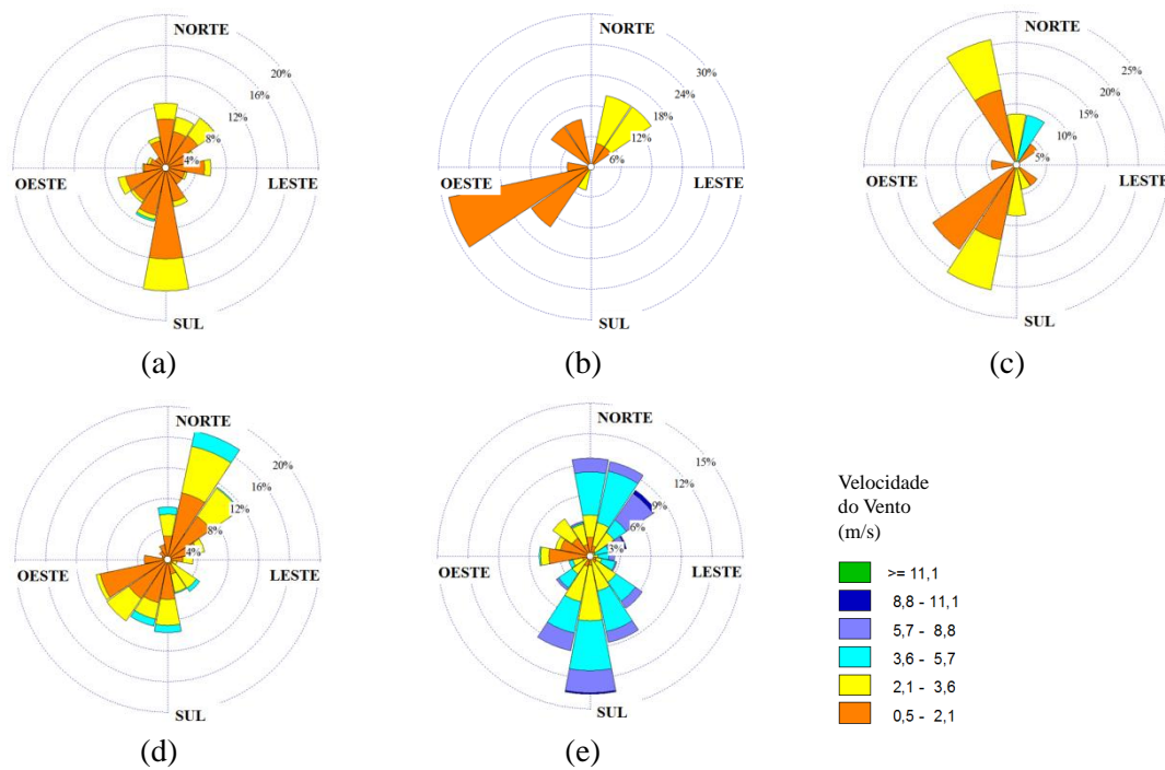
Figura 6.22. Rosa dos ventos para o mês de novembro nas estações: (a) Carapina, (b) Enseada do Suá, (c) Ibes, (d) Cariacica e (e) Aeroporto.
