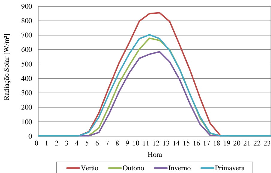
Figura 6.5. Radiação solar média horária nos períodos de solstício e equinócio na estação Carapina.
