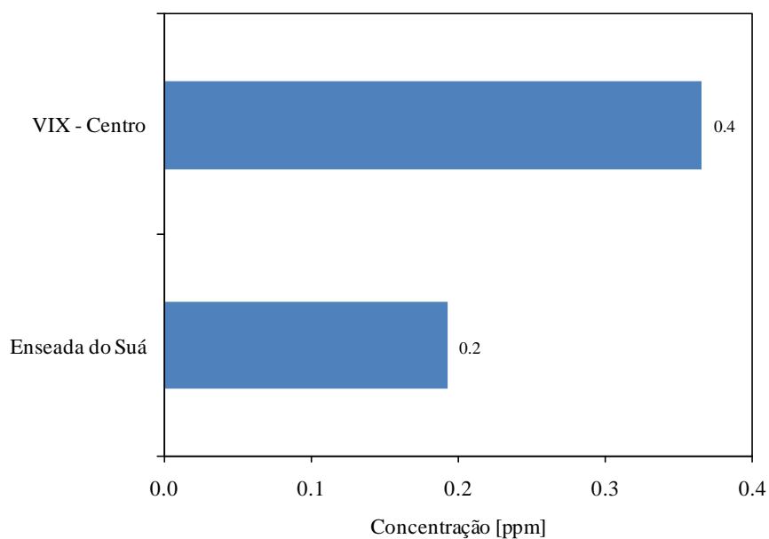
Figura 7.27. Concentração média anual de HCNM nas estações da RAMQAr (ano base 2012).
