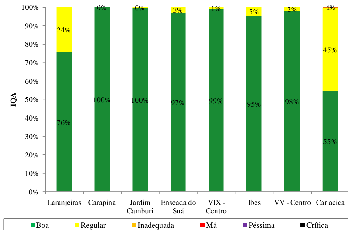
Figura 7.3. Índice de qualidade do ar com referência ao poluente MP_{10} nas estações da RAMQAr (ano base 2012).
