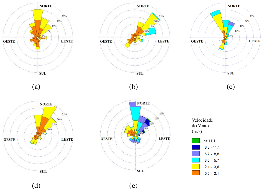
Figura 6.14. Rosa dos ventos para o mês de março nas estações: (a) Carapina; (b) Enseada do Suá; (c) Ibes; (d) Cariacica; e (e) Aeroporto.
