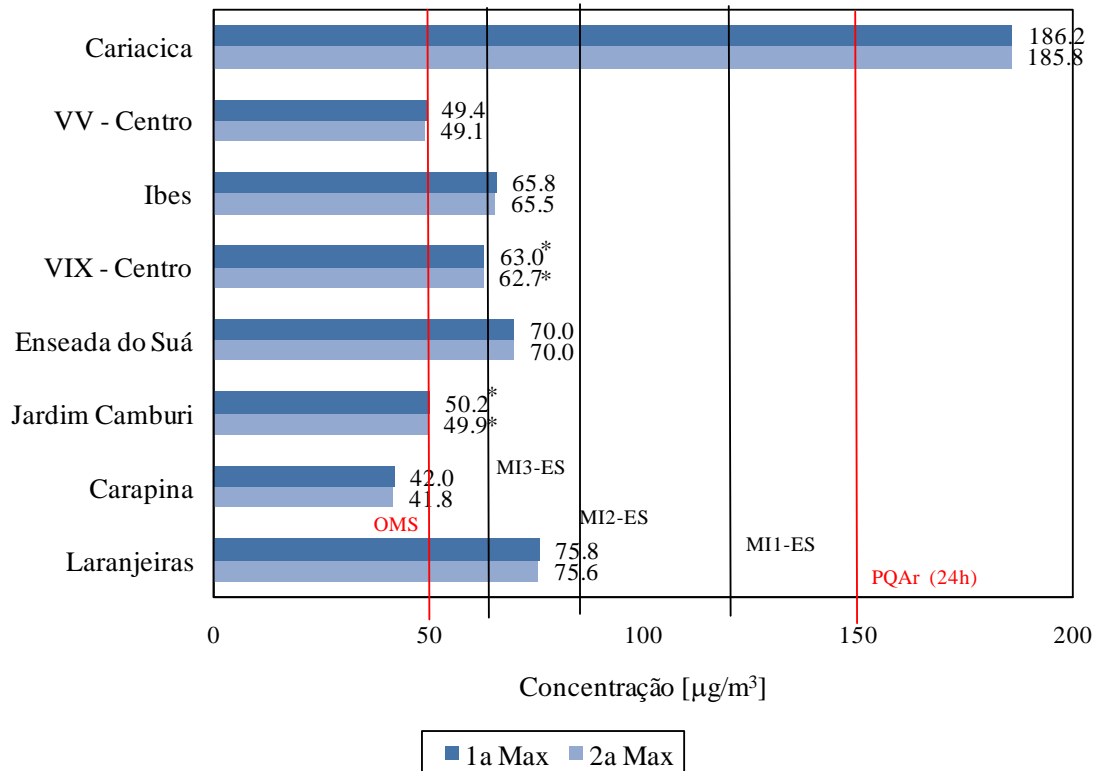
Figura 7.1. Concentração máxima média de 24h de MP_{10} nas estações da RAMQAr (ano base 2012). PQAr indica o padrão nacional de qualidade do ar. MI1-ES, MI2-ES e MI3-ES são as metas intermediárias. OMS representa a diretriz da Organização Mundial de Saúde para o referido poluente, que equivale ao padrão final preconizado na legislação estadual (PF-ES). Valores destacados com * são considerados não-representativos.
