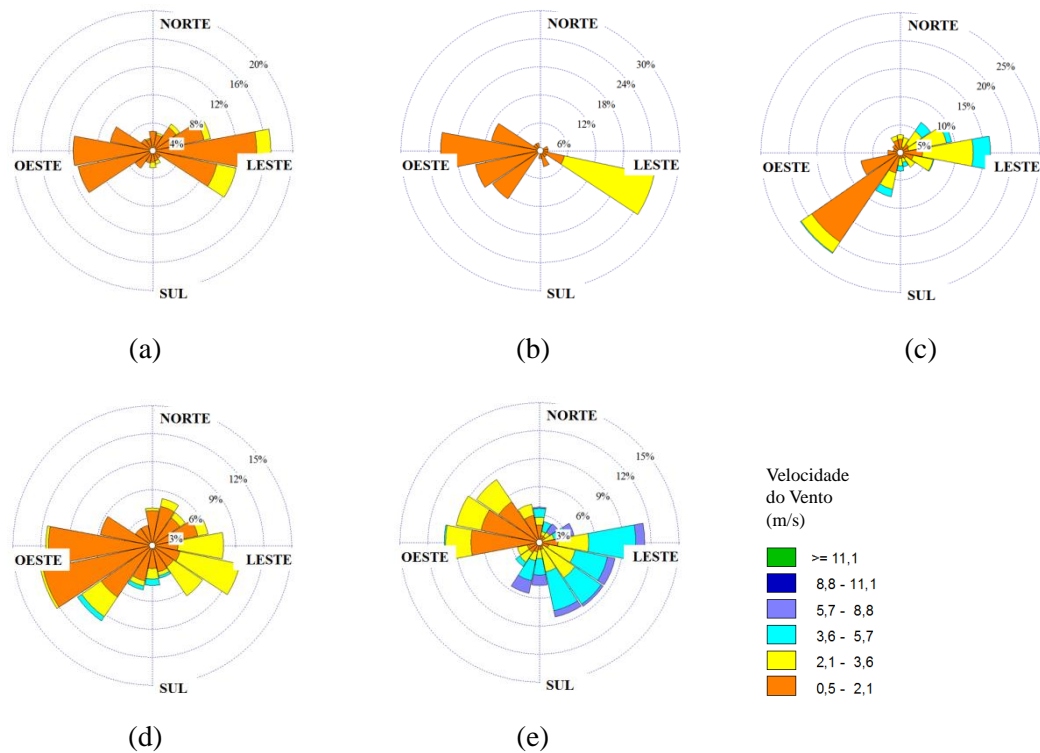
Figura 6.19. Rosa dos ventos para o mês de agosto nas estações: (a) Carapina; (b) Enseada do Suá; (c) Ibes; (d) Cariacica; e (e) Aeroporto.
