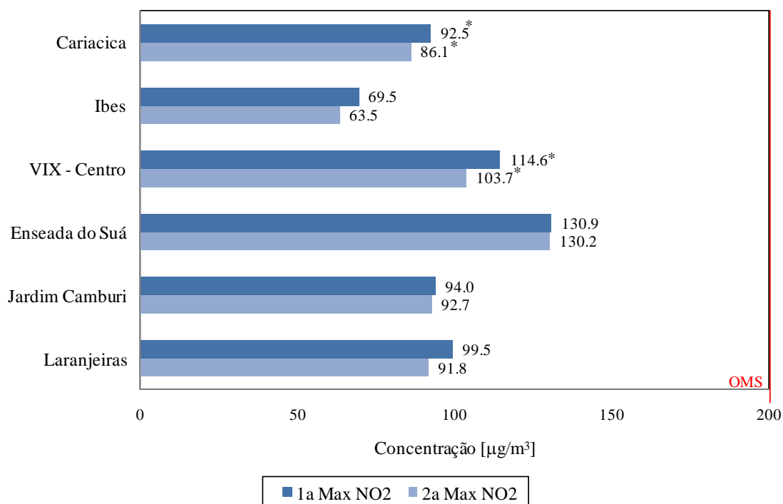
Figura 7.14. Concentrações horárias máximas de NO 2 nas estações da RAMQAr (ano base 2012). OMS representa a diretriz da Organização Mundial de Saúde para o referido poluente, que equivale ao padrão final preconizado na legislação estadual (PF-ES).
