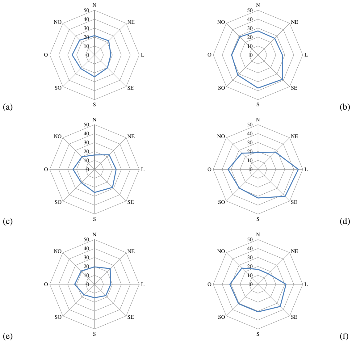
Figura 7.17. Perfil de concentração média horária de \text{NO}_2 nas estações da RAMQAr com relação à direção do vento (gráfico de radar):(a) Laranjeiras**; (b) Jardim Camburi**; (c) Enseada do Suá; (d) VIX-Centro**; (e) Ibes; e (f) Cariacica**.
