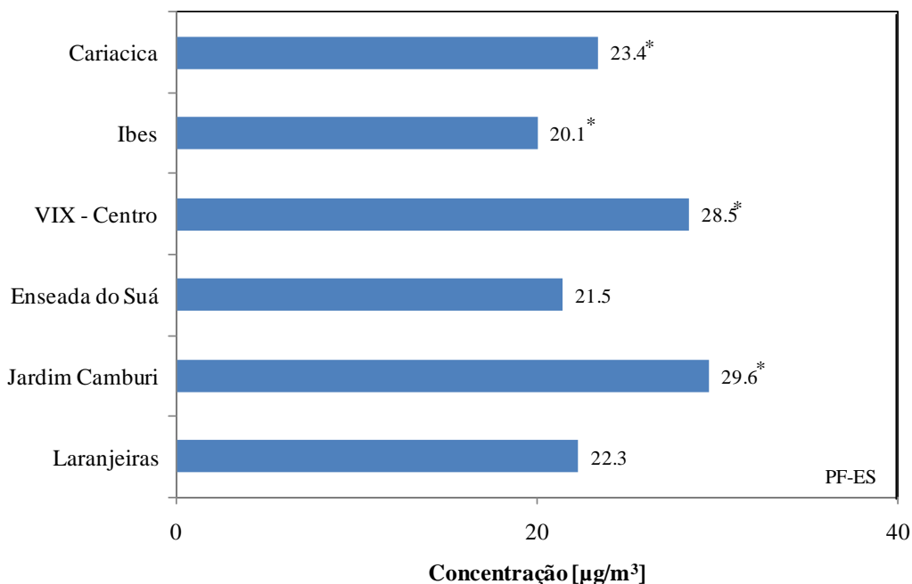
Figura 7.15. Concentrações médias anuais de NO 2 nas estações da RAMQAr (ano base 2012). PF-ES é o padrão final preconizado na legislação estadual.
