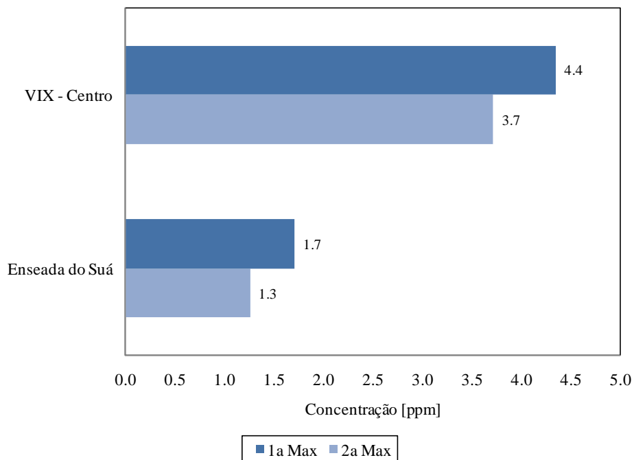
Figura 7.26. Concentração diária máxima de HCNM nas estações da RAMQAr (ano base 2012).
