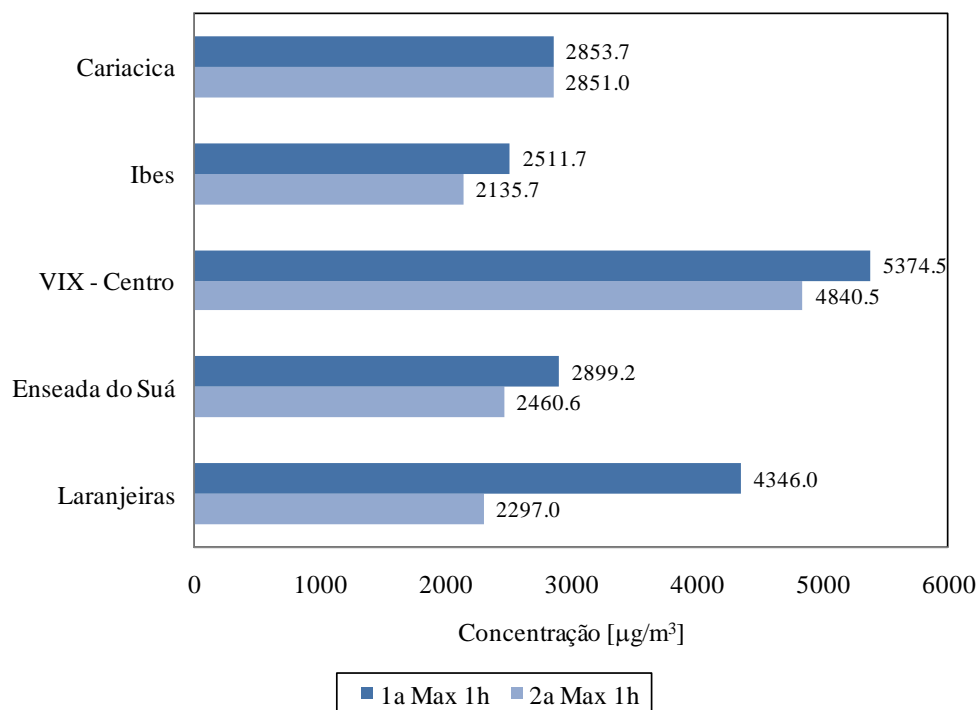
Figura 7.23. Concentração horária máxima de CO nas estações da RAMQAr (ano base 2012).
