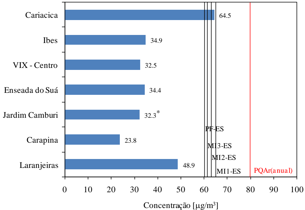
Figura 7.6. Concentração média anual de PTS nas estações da RAMQAr (ano base 2012). PQAr indica o padrão nacional de qualidade do ar. MI1-ES, MI2-ES e MI3-ES são as metas intermediárias e PF-ES é o padrão final preconizado na legislação estadual. Valores destacados com * são considerados não-representativos.
