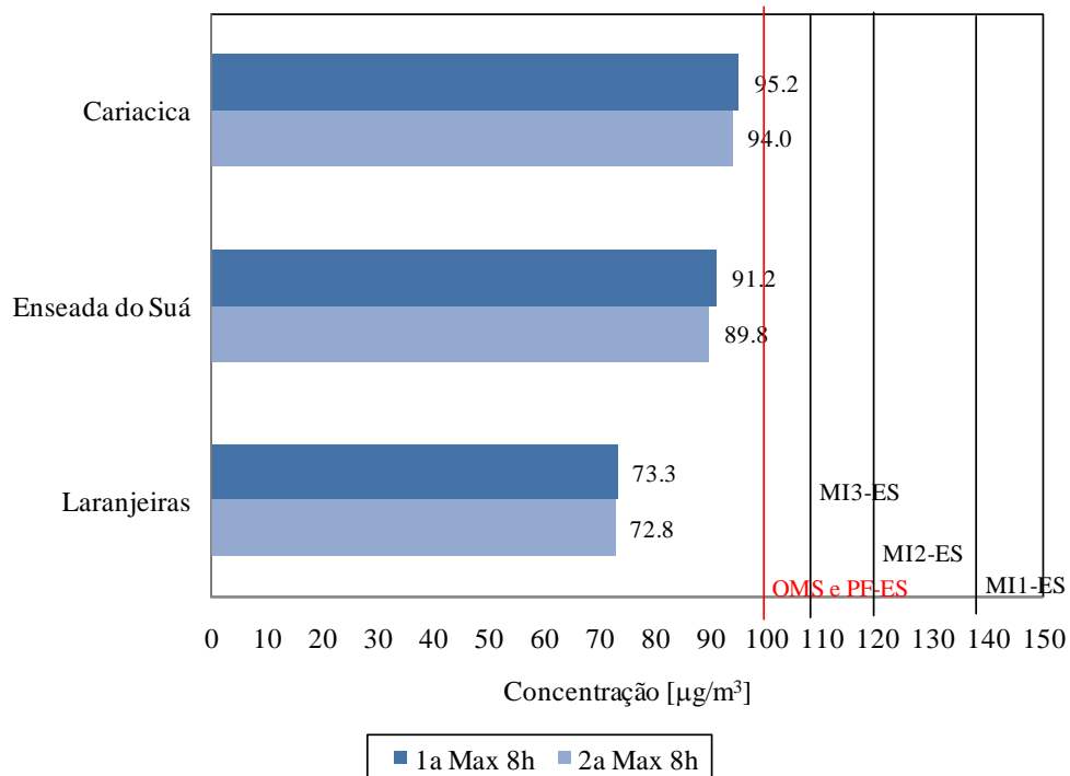
Figura 7.18. Concentração média 8h máxima de O 3 nas estações da RAMQAr (ano base 2012). PQAr indica o padrão nacional de qualidade do ar. MI1-ES, MI2-ES e MI3-ES são as metas intermediárias. OMS representa a diretriz da Organização Mundial de Saúde para o referido poluente, que equivale ao padrão final preconizado na legislação estadual (PF-ES). Valores destacados com * são considerados não-representativos.
