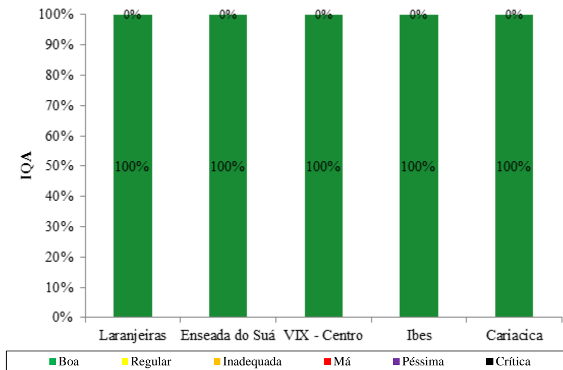
Figura 7.24. Índice de qualidade do ar com referência ao poluente CO nas estações da RAMQAr (ano base 2012).
