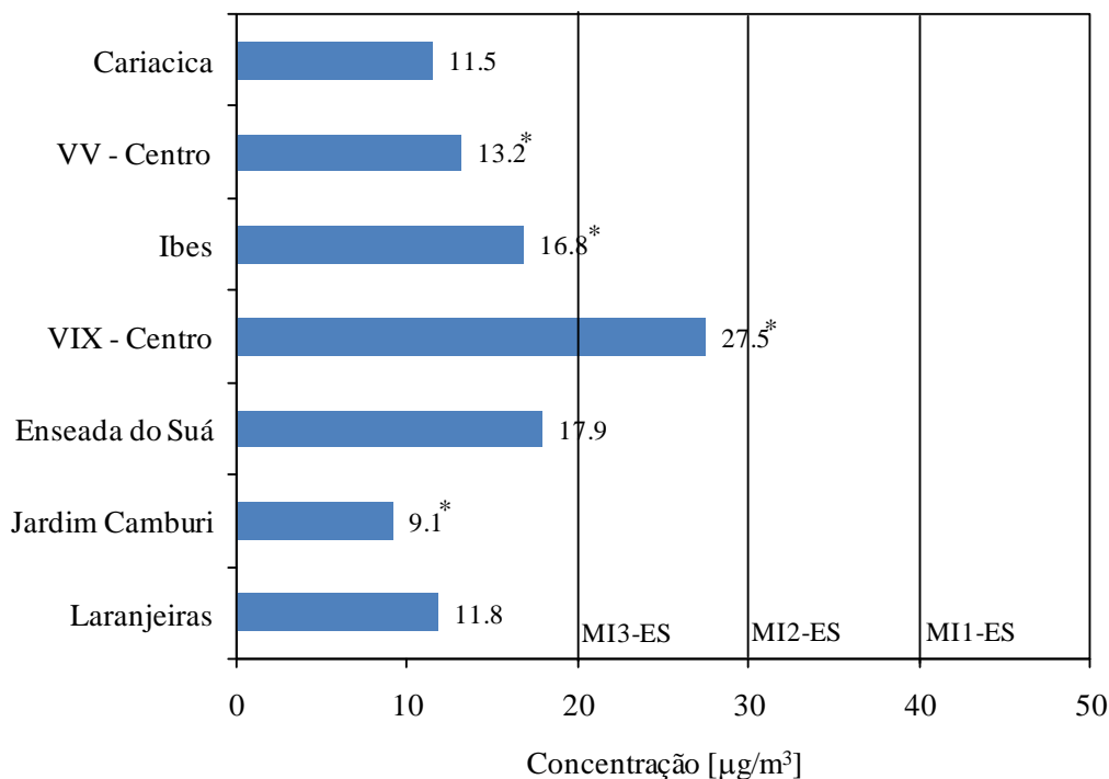
Figura 7.11. Concentração média anual de \text{SO}_2 nas estações da RAMQAr (ano base 2012). PQAr indica o padrão nacional de qualidade do ar. MI1-ES, MI2-ES e MI3-ES são as metas intermediárias. Valores destacados com * são considerados não-representativos.
