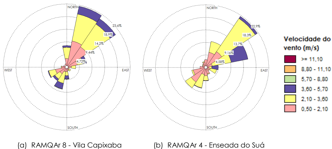
Gráfico 5.19 - Rosa dos ventos para o mês de setembro na RMGV.
