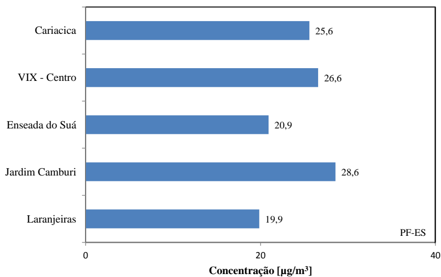
Figura 7.21. Concentrações médias anuais de NO_2 nas estações da RAMQAr (ano base 2013). PF-ES é o padrão final preconizado na legislação estadual.
