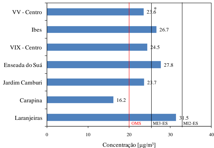
Figura 7.2. Concentração média anual de MP_{10} nas estações da RAMQAr (ano base 2013). PQAr indica o padrão nacional de qualidade do ar. MI1-ES, MI2-ES e MI3-ES são as metas intermediárias. OMS representa a diretriz da Organização Mundial de Saúde para o referido poluente, que equivale ao padrão final preconizado na legislação estadual (PF-ES). Valores destacados com * são considerados não-representativos.
