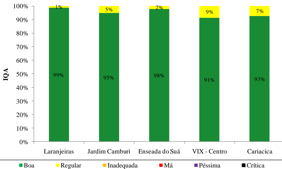
Figura 7.22. Índice de qualidade do ar referente ao poluente NO 2 nas estações da RAMQAr (ano base 2013).
