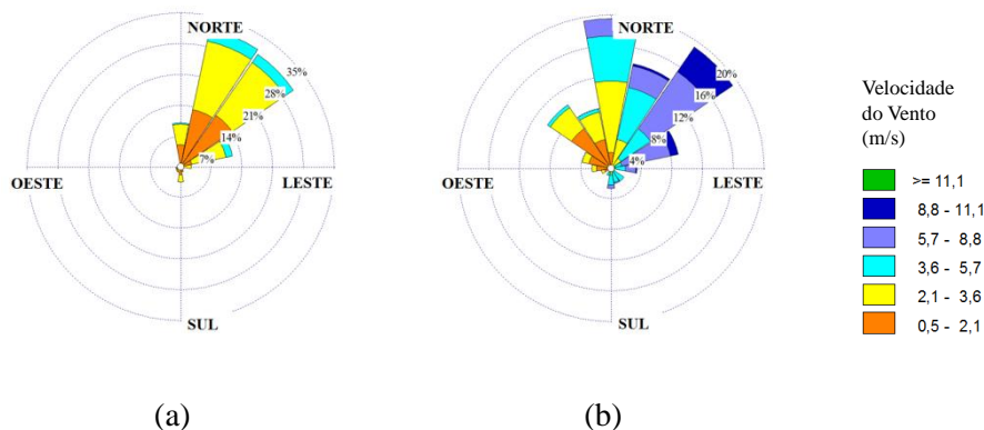
Figura 6.13. Rosa dos ventos para o mês de fevereiro nas estações: (a) Cariacica e (b) Aeroporto.
