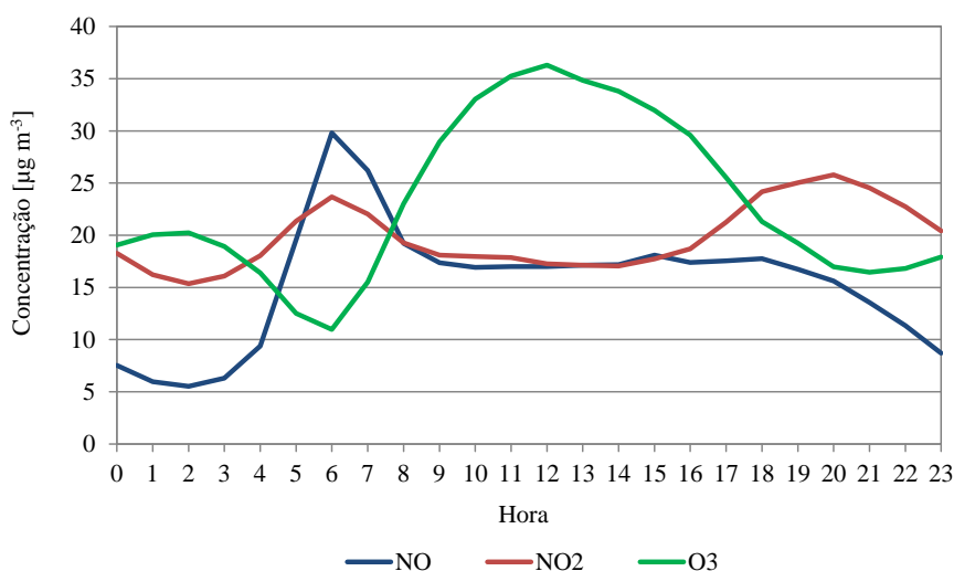
Figura 7.29. Evolução horária dos poluentes monóxido de nitrogênio (NO), dióxido de nitrogênio ( NO_2 ) e ozônio ( O_3 ) na Estação Laranjeiras para o ano de 2013.
