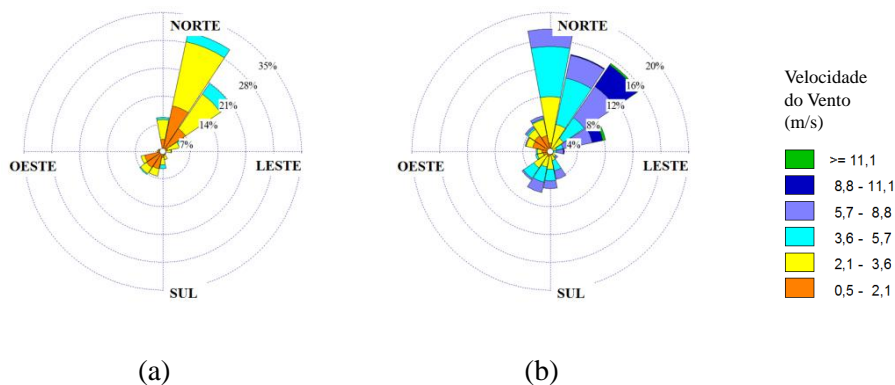
Figura 6.12. Rosa dos ventos para o mês de janeiro nas estações: (a) Cariacica e (b) Aeroporto.
