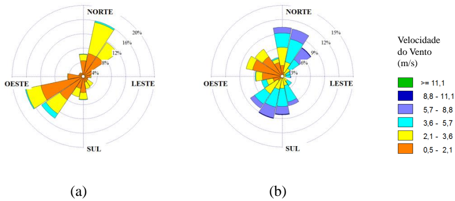
Figura 6.18. Rosa dos ventos para o mês de julho nas estações: (a) Cariacica e (b) Aeroporto.
