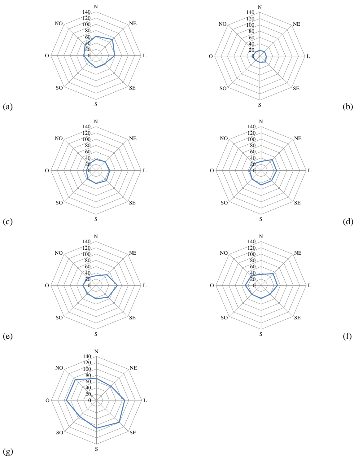
Figura 7.10. Perfil de concentração média horária de PTS nas estações da RAMQAr com relação à direção do vento (gráfico de radar)**: (a) Laranjeiras; (b) Carapina; (c) Jardim Camburi; (d) Enseada do Suá; (e) VIX-Centro; (f) Ibes e (g) Cariacica.
