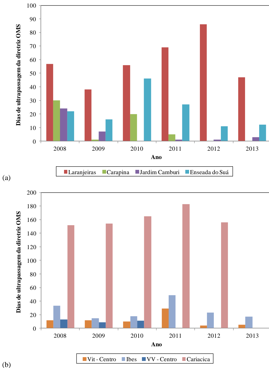
Figura 7.6. Número de dias de ultrapassagem da diretriz da OMS para o poluente MP_{10} (curta exposição) entre os anos 2008 e 2013 nas estações (a) Laranjeiras, Carapina, Jardim Camburi, Enseada do Suá, VIX-Centro e (b) Ibes, VV-Centro e Cariacica.
