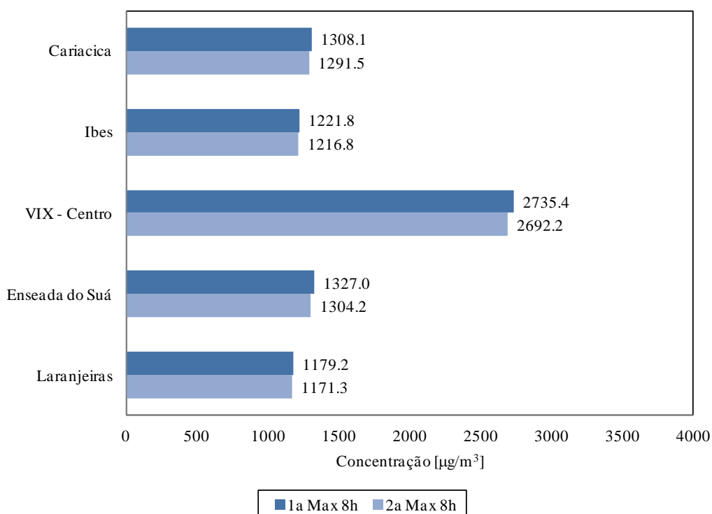
Figura 7.30. Concentração média de 8h máxima de CO nas estações da RAMQAr (ano base 2013).
