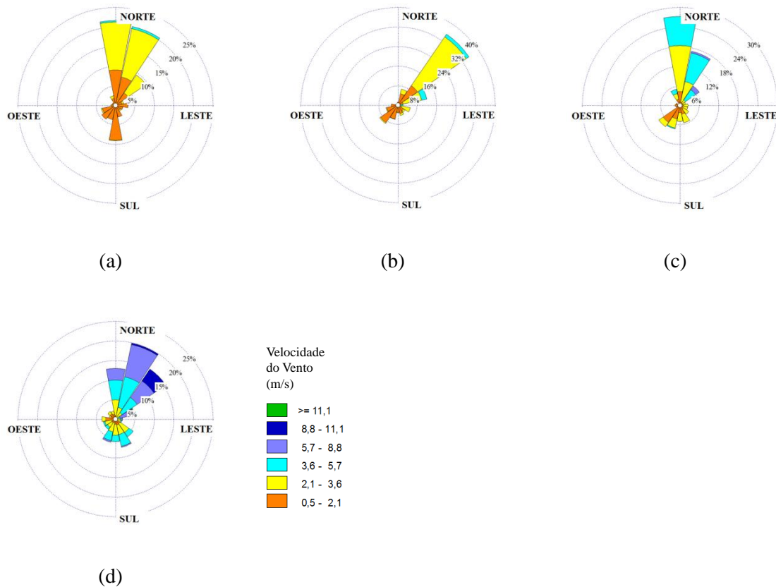
Figura 6.23. Rosa dos ventos para o mês de dezembro nas estações: (a) Carapina, (b) Enseada do Suá, (c) Ibes e (d) Aeroporto.
