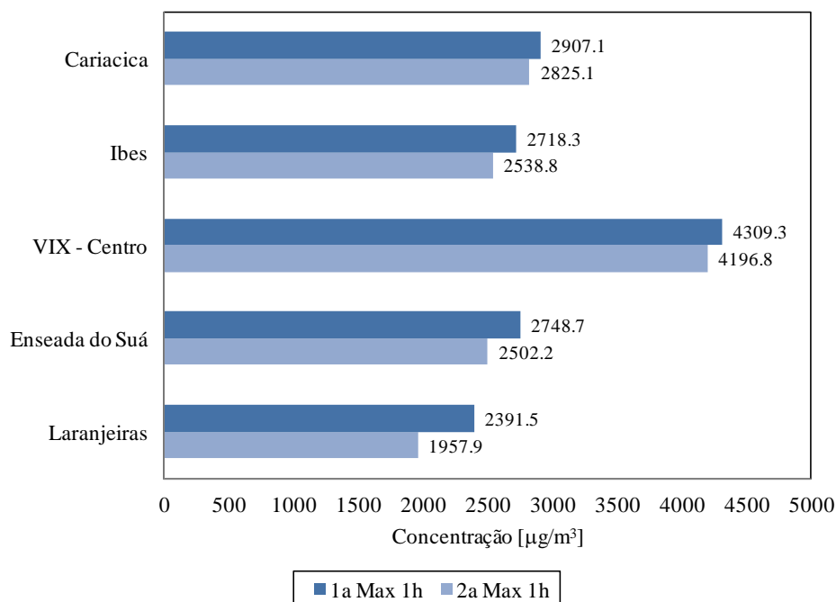
Figura 7.31. Concentração horária máxima de CO nas estações da RAMQAr (ano base 2013).
