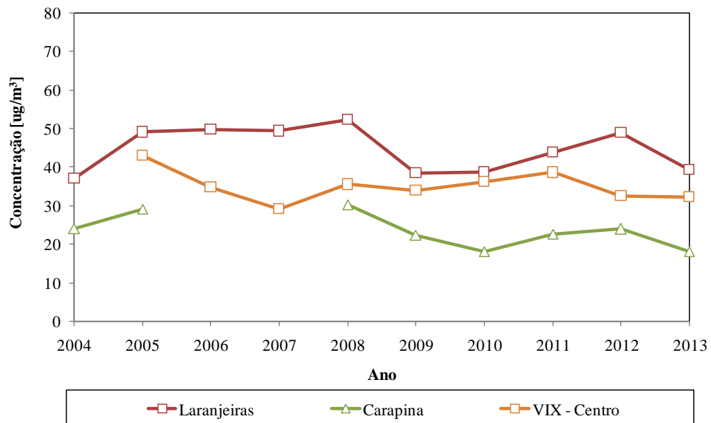
Figura 7.11. Séries temporais das concentrações médias anuais de PTS nas estações da RAMQAr.
