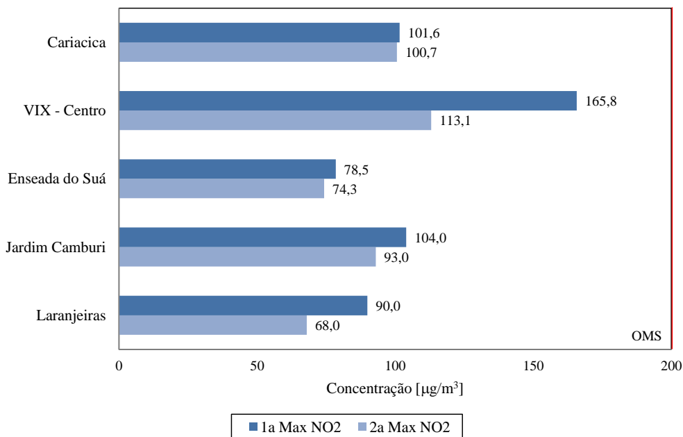
Figura 7.20. Concentrações horária máximas de NO_2 nas estações da RAMQAr (ano base 2013). OMS representa a diretriz da Organização Mundial de Saúde para o referido poluente, que equivale ao padrão final preconizado na legislação estadual (PF-ES).
