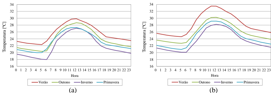
Figura 6.3. Temperatura média horária por estações do ano nas estações: (a) Carapina e (b) Cariacica.
