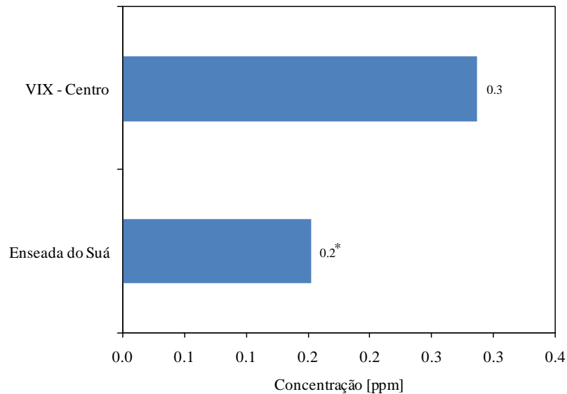
Figura 7.35. Concentração média anual de HCNM nas estações da RAMQAr (ano base 2013).
