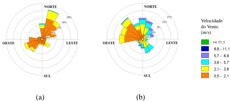
Figura 6.17. Rosa dos ventos para o mês de junho nas estações: (a) Cariacica e (b) Aeroporto.
