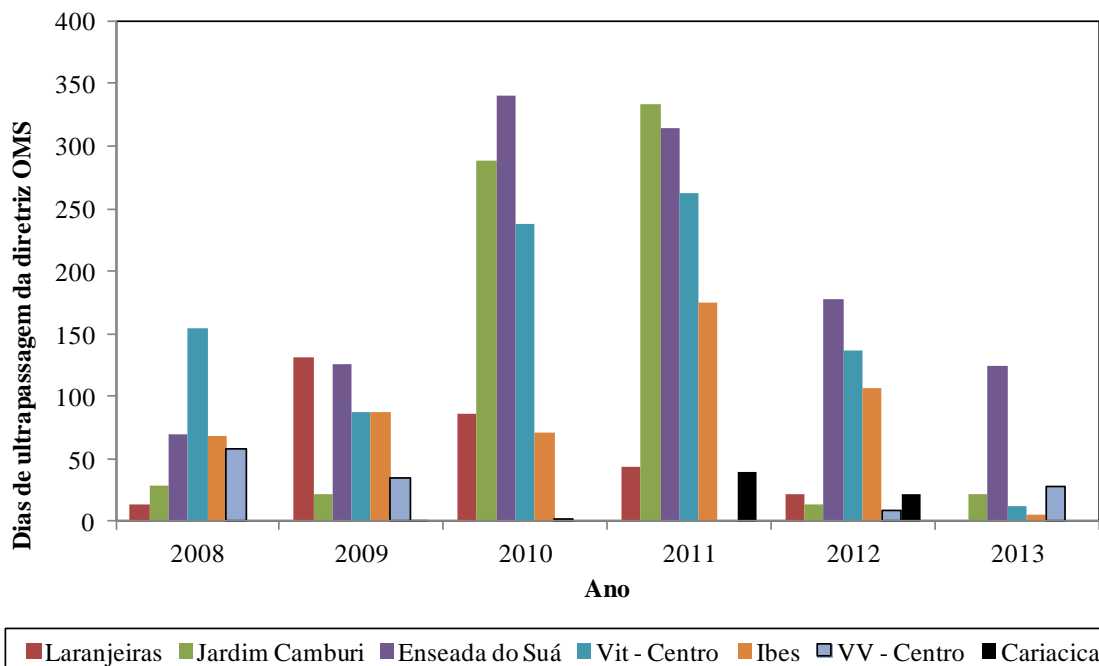
Figura 7.19. Número de dias de ultrapassagens da diretriz da OMS (idêntico ao do padrão final da legislação estadual) para o poluente SO 2 entre 2008 e 2013.
