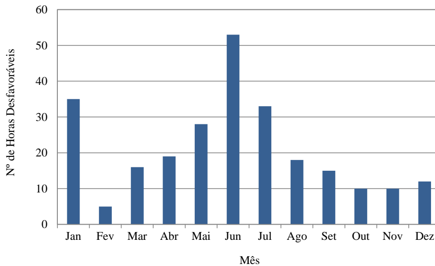
Figura 6.24. Número de horas desfavoráveis à dispersão de poluentes.
