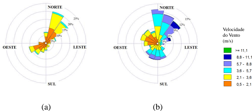
Figura 6.10. Rosa dos ventos anual nas estações: (a) Cariacica e (b) Aeroporto.
