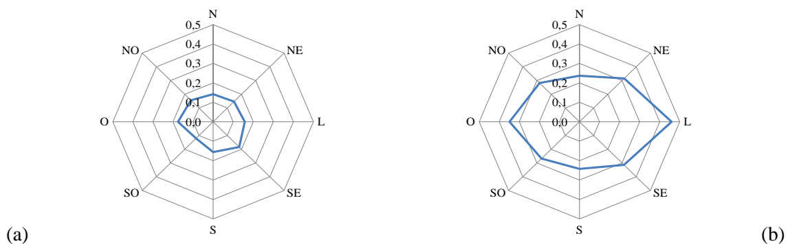
Figura 7.36. Perfil de concentração média horária de HCNM nas estações da RAMQAr com relação à direção do vento**: (a) Enseada do Suá e (b) VIX-Centro.
