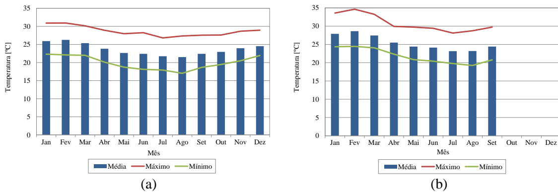
Figura 6.2. Temperatura média mensal, máxima e mínima nas estações: (a) Carapina e (b) Cariacica.
