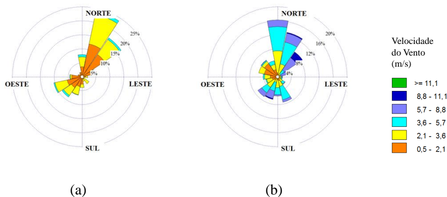
Figura 6.14. Rosa dos ventos para o mês de março nas estações: (a) Cariacica e (b) Aeroporto.
