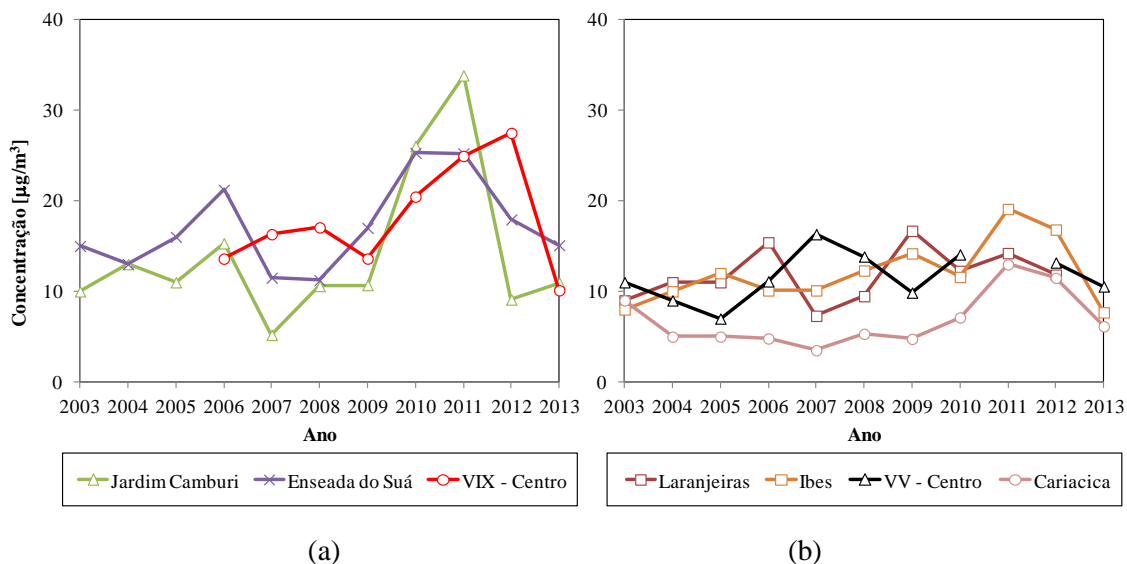
Figura 7.18. Séries temporais das concentrações médias anuais de SO 2 nas estações da RAMQAr.
