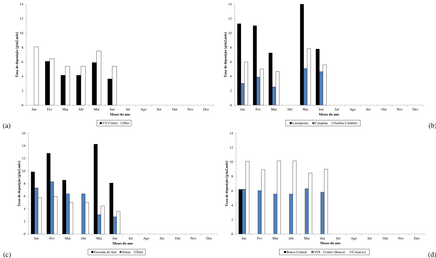
Figura 7.12. Taxa de deposição de partículas (g/m 2 /30 dias) nas estações de monitoramento de PS (ano base 2013).
