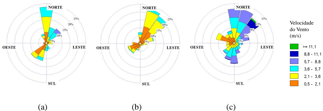
Figura 6.20. Rosa dos ventos para o mês de setembro nas Estações: (a) Ibes, (b) Cariacica; e (c) Aeroporto.
