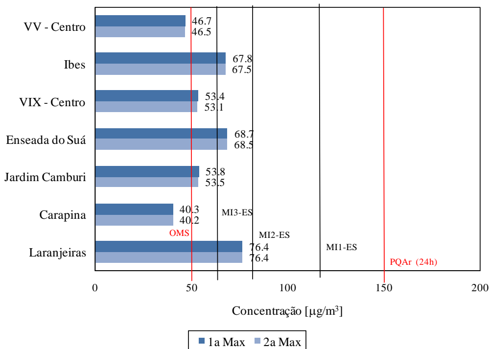
Figura 7.1. Concentração máxima média de 24h de MP_{10} nas estações da RAMQAr (ano base 2013). PQAr indica o padrão nacional de qualidade do ar. MI1-ES, MI2-ES e MI3-ES são as metas intermediárias. OMS representa a diretriz da Organização Mundial de Saúde para o referido poluente, que equivale ao padrão final preconizado na legislação estadual (PF-ES). Valores destacados com * são considerados não-representativos.
