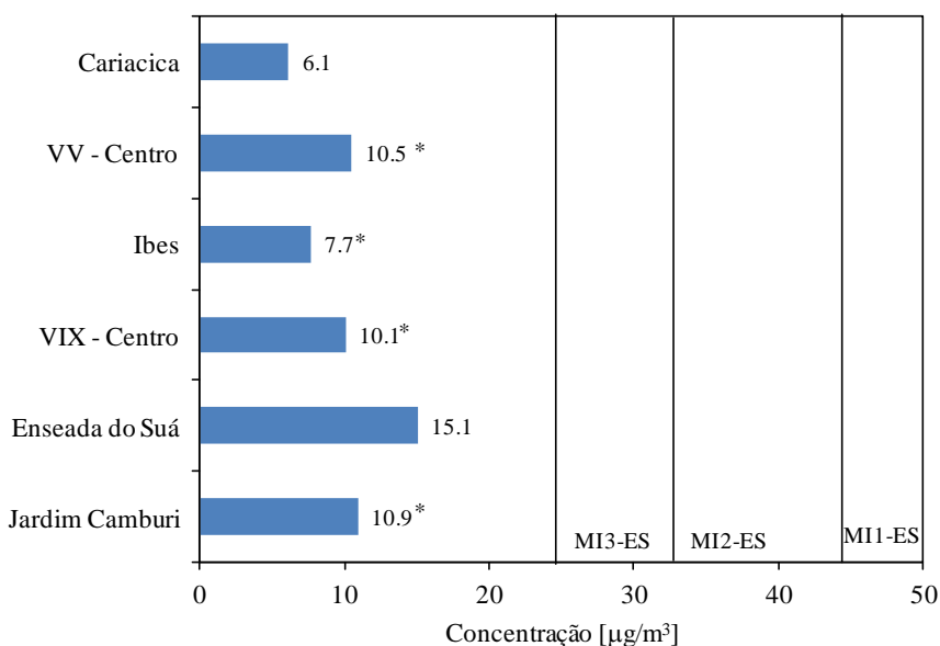
Figura 7.15. Concentração média anual de SO 2 nas estações da RAMQAr (ano base 2013). PQAr indica o padrão nacional de qualidade do ar. MI1-ES, MI2-ES e MI3-ES são as metas intermediárias. Valores destacados com * são considerados não-representativos.
