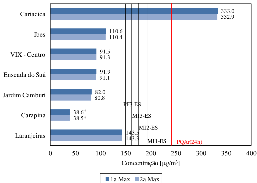
Figura 7.7. Concentração máxima média de 24h de PTS nas estações da RAMQAr (ano base 2013). PQAr indica o padrão nacional de qualidade do ar. MI1-ES, MI2-ES e MI3-ES são as metas intermediárias e PF-ES é o padrão final preconizado na legislação estadual. Valores destacados com * são considerados não-representativos.
