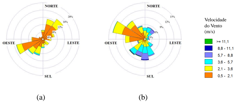
Figura 6.16. Rosa dos ventos para o mês de maio nas estações: (a) Cariacica e (b) Aeroporto.
