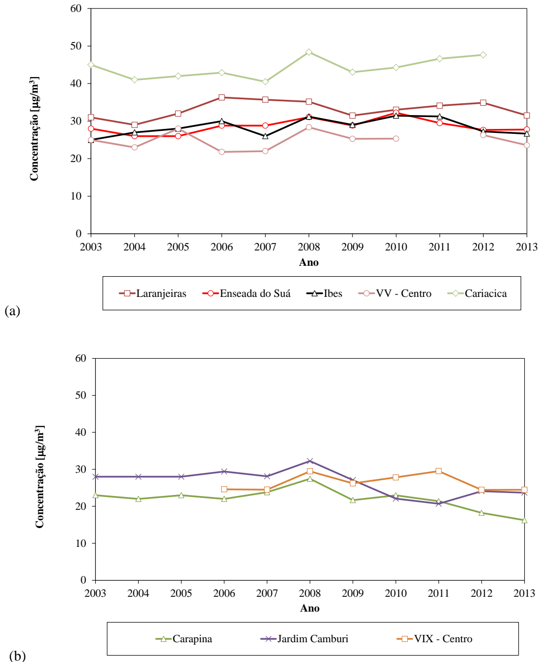
Figura 7.5. Séries temporais das concentrações médias anuais de PM_{10} nas estações da RAMQAr.
