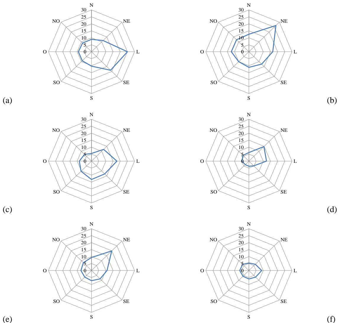
Figura 7.17. Perfil de concentração média horária de \text{SO}_2 nas estações da RAMQAr com relação à direção do vento (gráfico de radar)**: (a) Jardim Camburi; (b) Enseada do Suá; (c) VIX-Centro; (d) Ibes; (e) VV-Centro e (f) Cariacica.
