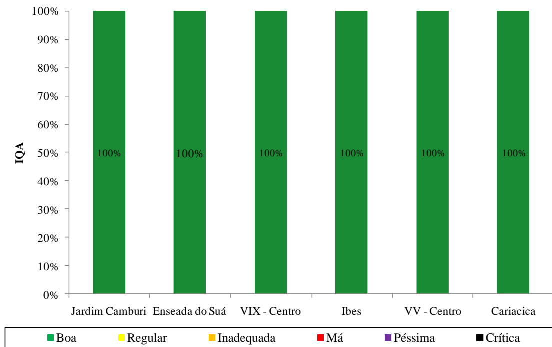
Figura 7.16. Índice de qualidade do ar com referência ao poluente SO 2 nas estações da RAMQAr (ano base 2013).
