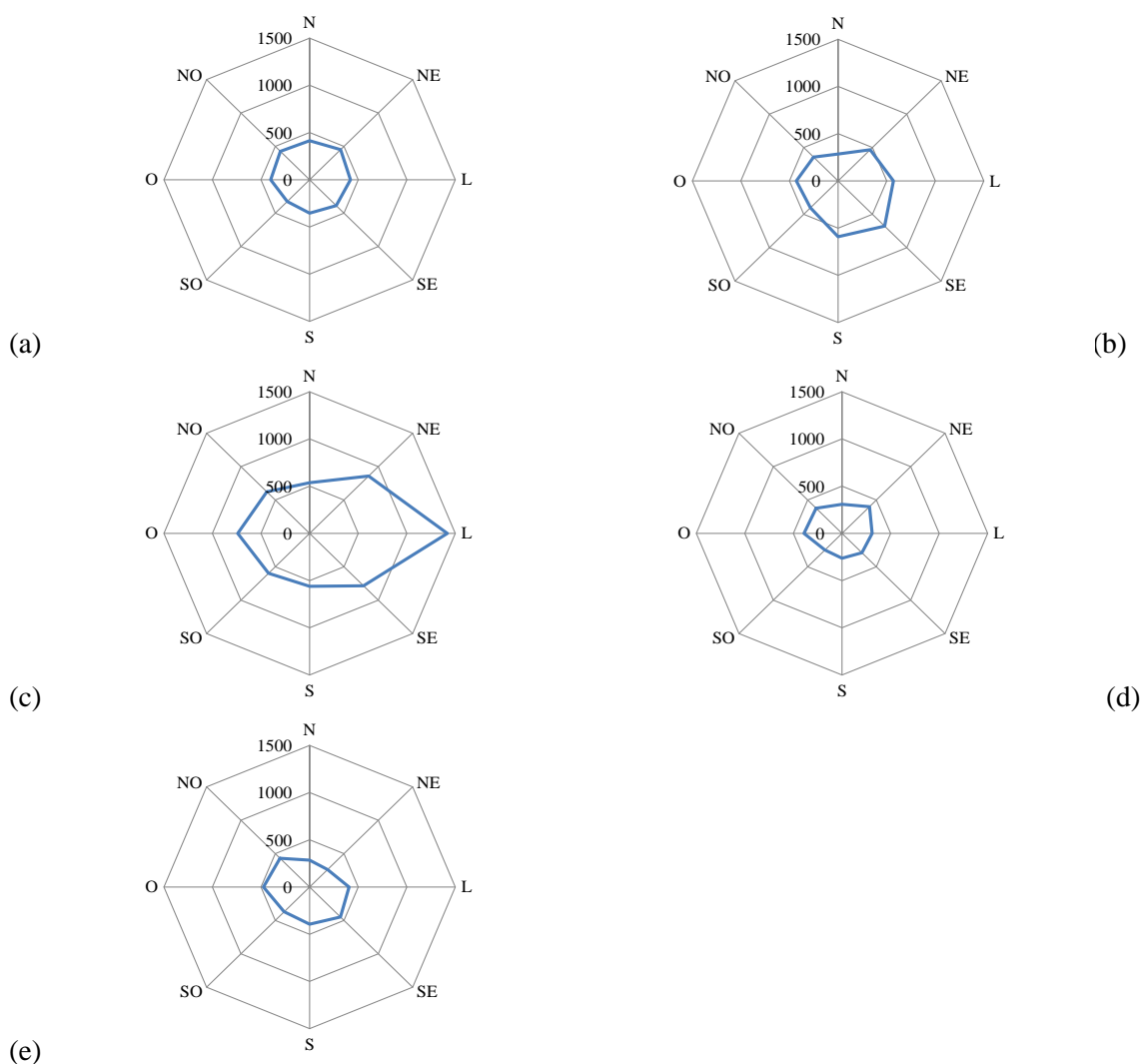
Figura 7.33. Perfil de concentração média horária de CO nas estações da RAMQAr com relação à direção do vento (gráfico de radar): (a) Laranjeiras**;
