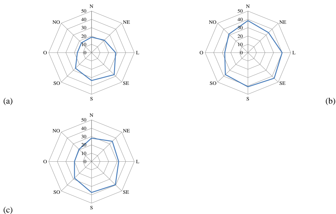
Figura 7.28. Perfil de concentração média horária de O_3 nas estações da RAMQAr com relação à direção do vento (gráfico de radar)**: (a) Laranjeiras; (b) Enseada do Suá e (c) Cariacica.
