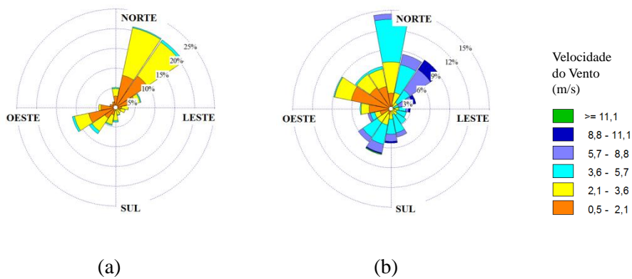
Figura 6.19. Rosa dos ventos para o mês de agosto nas estações: (a) Cariacica e (b) Aeroporto.
