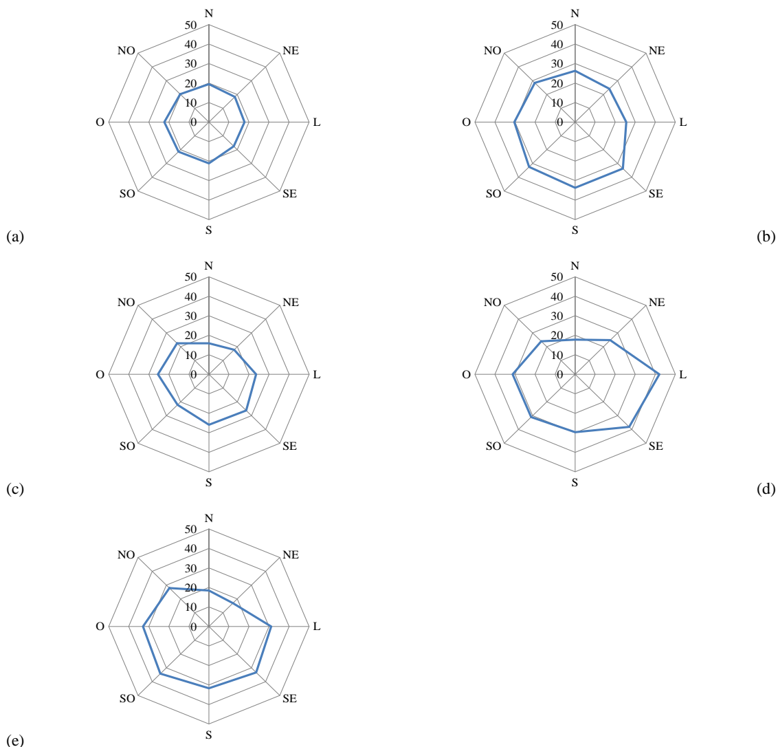
Figura 7.23. Perfil de concentração média horária de \text{NO}_2 nas estações da RAMQAr com relação à direção do vento (gráfico de radar)**: (a) Laranjeiras; (b) Jardim Camburi; (c) Enseada do Suá; (d) VIX-Centro e (e) Cariacica.
