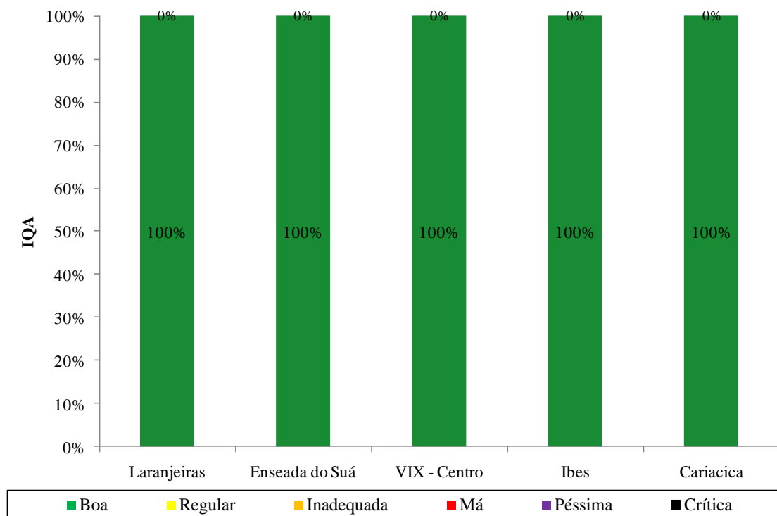
Figura 7.32. Índice de qualidade do ar com referência ao poluente CO nas estações da RAMQAr (ano base 2013).
