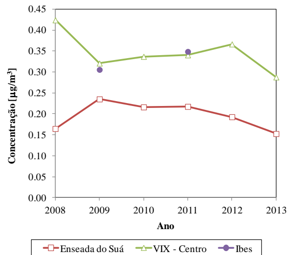
Figura7.37. Séries temporais das concentrações médias anuais de HCNM nas estações da RAMQAr.
