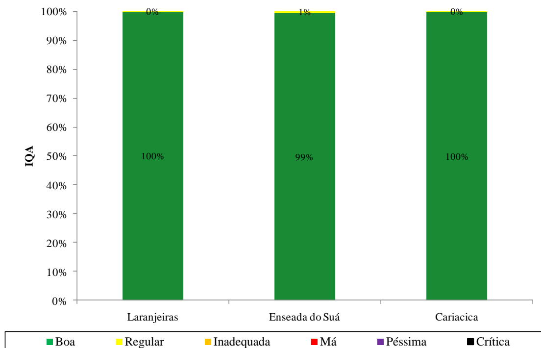
Figura 7.27. Índice de qualidade do ar com referência ao poluente O_3 nas estações da RAMQAr (ano base 2013).
