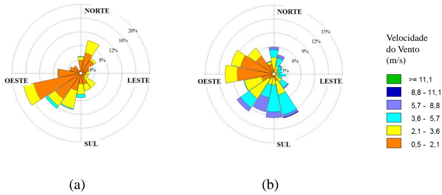
Figura 6.15. Rosa dos ventos para o mês de abril nas estações: (a) Cariacica e (b) Aeroporto.
