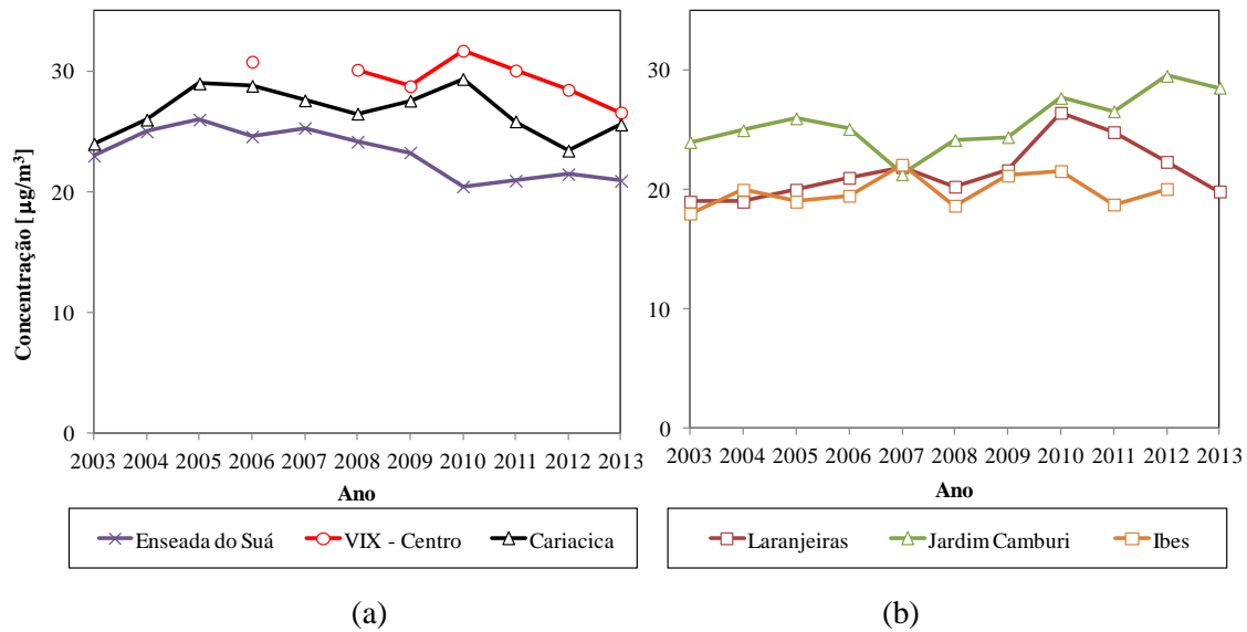
Figura 7.24. Séries temporais das concentrações médias anuais de \text{NO}_2 nas estações da RAMQAr.
