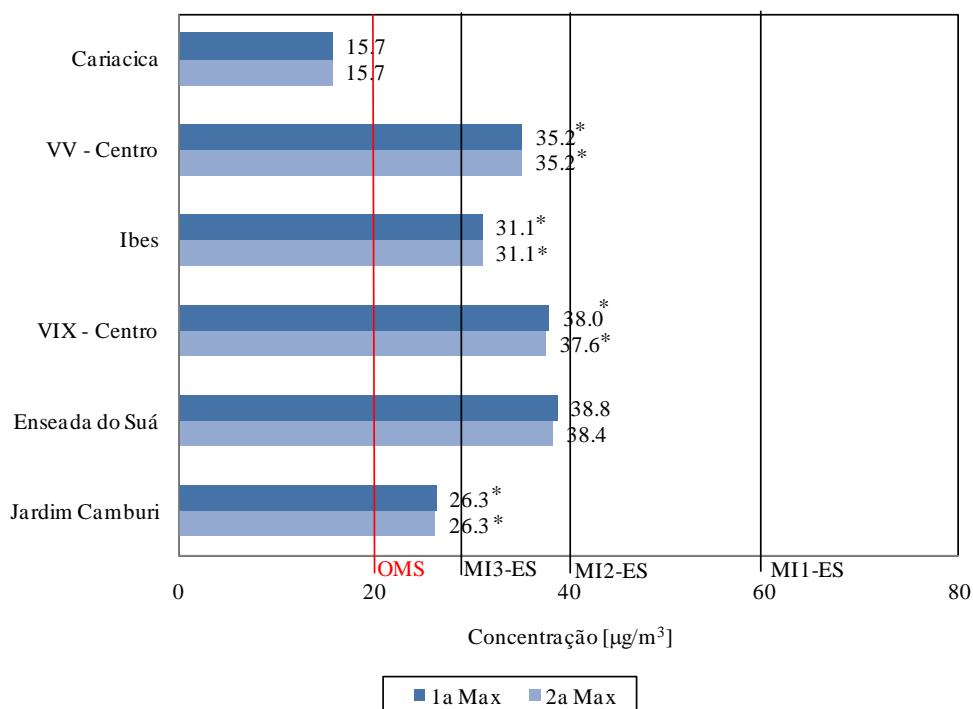
Figura 7.14. Concentração diária máxima de SO 2 nas estações da RAMQAr (ano base 2013). PQAr indica o padrão nacional de qualidade do ar. MI1-ES, MI2-ES e MI3-ES são as metas intermediárias. OMS representa a diretriz da Organização Mundial de Saúde para o referido poluente, que equivale ao padrão final preconizado na legislação estadual (PF-ES). Valores destacados com * são considerados não-representativos.
