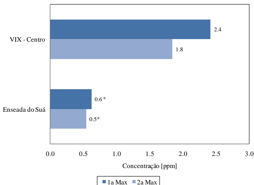
Figura 7.34. Concentração diária máxima de HCNM nas estações da RAMQAr (ano base 2013). Valores destacados com * são considerados não-representativos.
