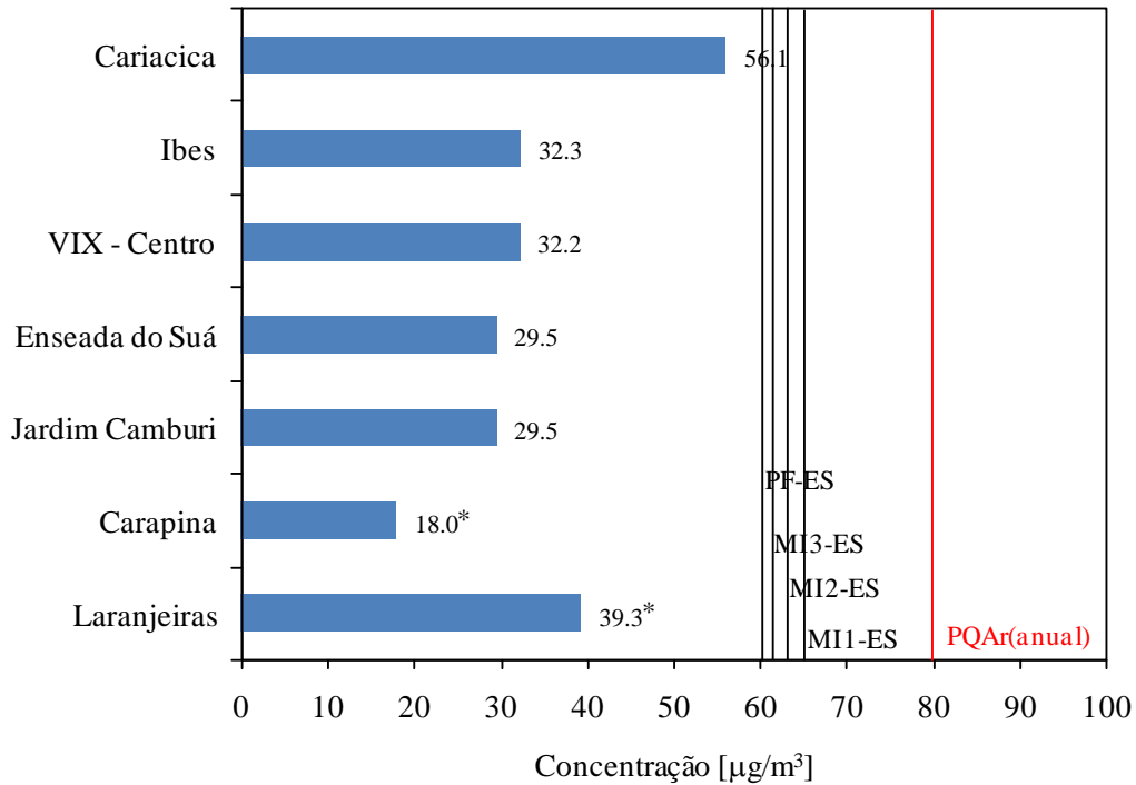
Figura 7.8. Concentração média anual de PTS nas estações da RAMQAr (ano base 2013). PQAr indica o padrão nacional de qualidade do ar. MI1-ES, MI2-ES e MI3-ES são as metas intermediárias e PF-ES é o padrão final preconizado na legislação estadual. Valores destacados com * são considerados não-representativos.
