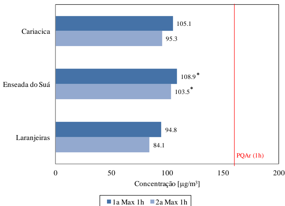
Figura 7.26. Concentração horária máxima de O_3 nas estações da RAMQAr (ano base 2013). PQAr indica o padrão nacional de qualidade do ar. Valores destacados com * são considerados não-representativos.
