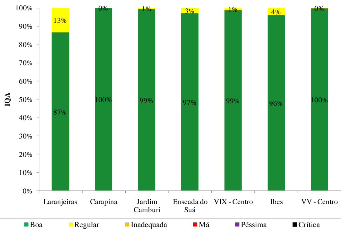
Figura 7.3. Índice de qualidade do ar com referência ao poluente MP_{10} nas estações da RAMQAr (ano base 2013).
