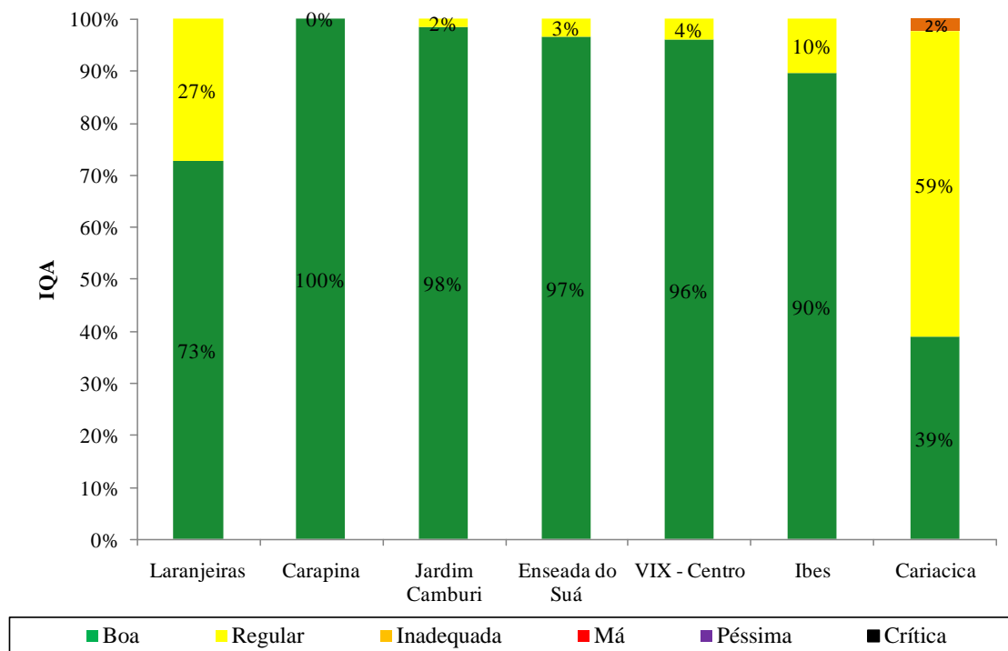
Figura 7.9. Índice de qualidade do ar com base no poluente PTS nas estações da RAMQAr (ano base 2013).
