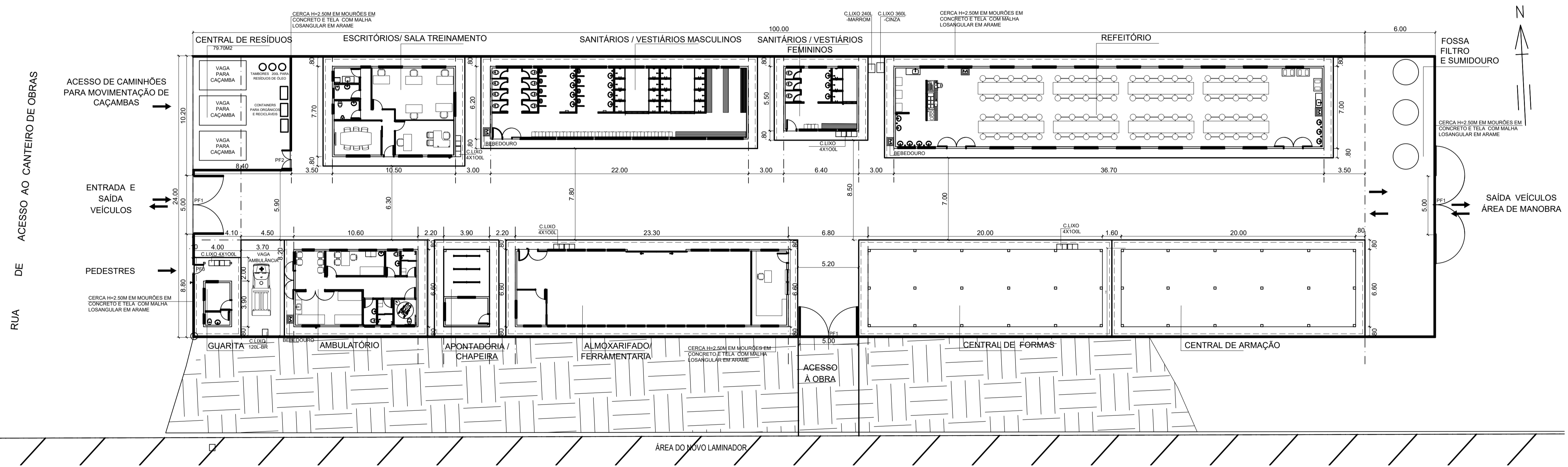
IMPLANTAÇÃO GERAL-PLANTA BAIXA ESC.:1:200
