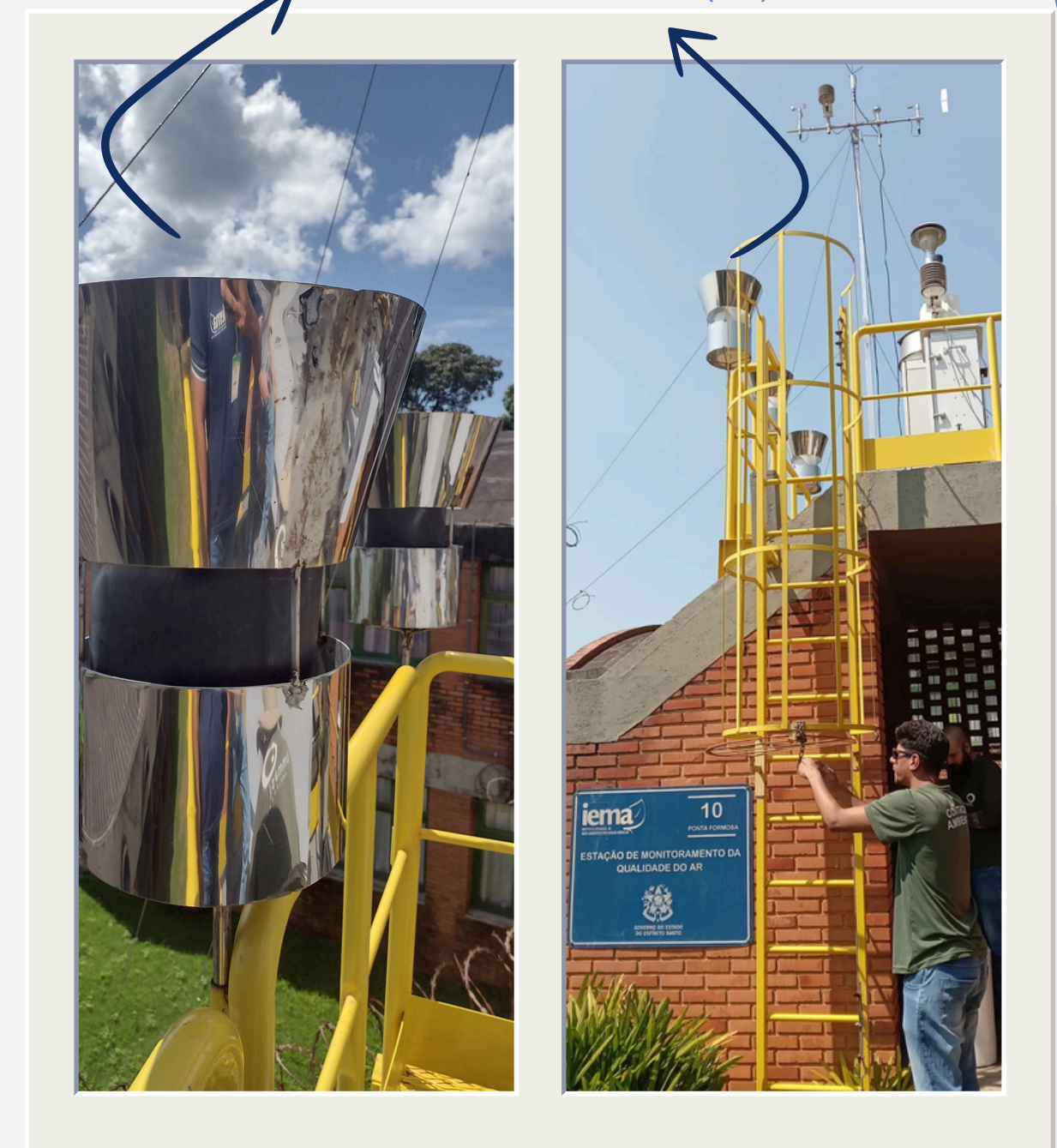
Recipiente coletor de Partícula Sedimentável (PS)
